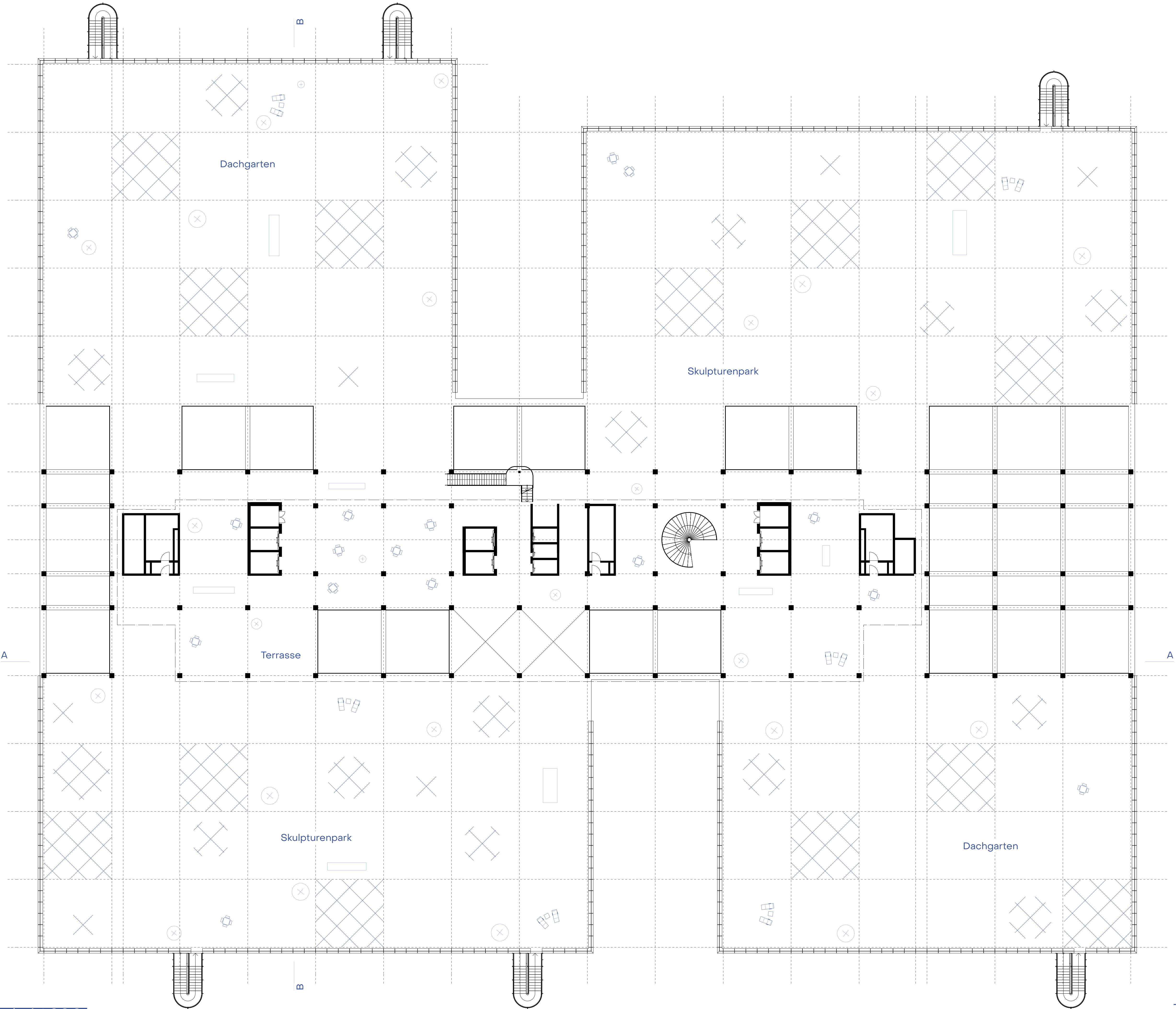
Dachgeschoss Sockel 1:200
