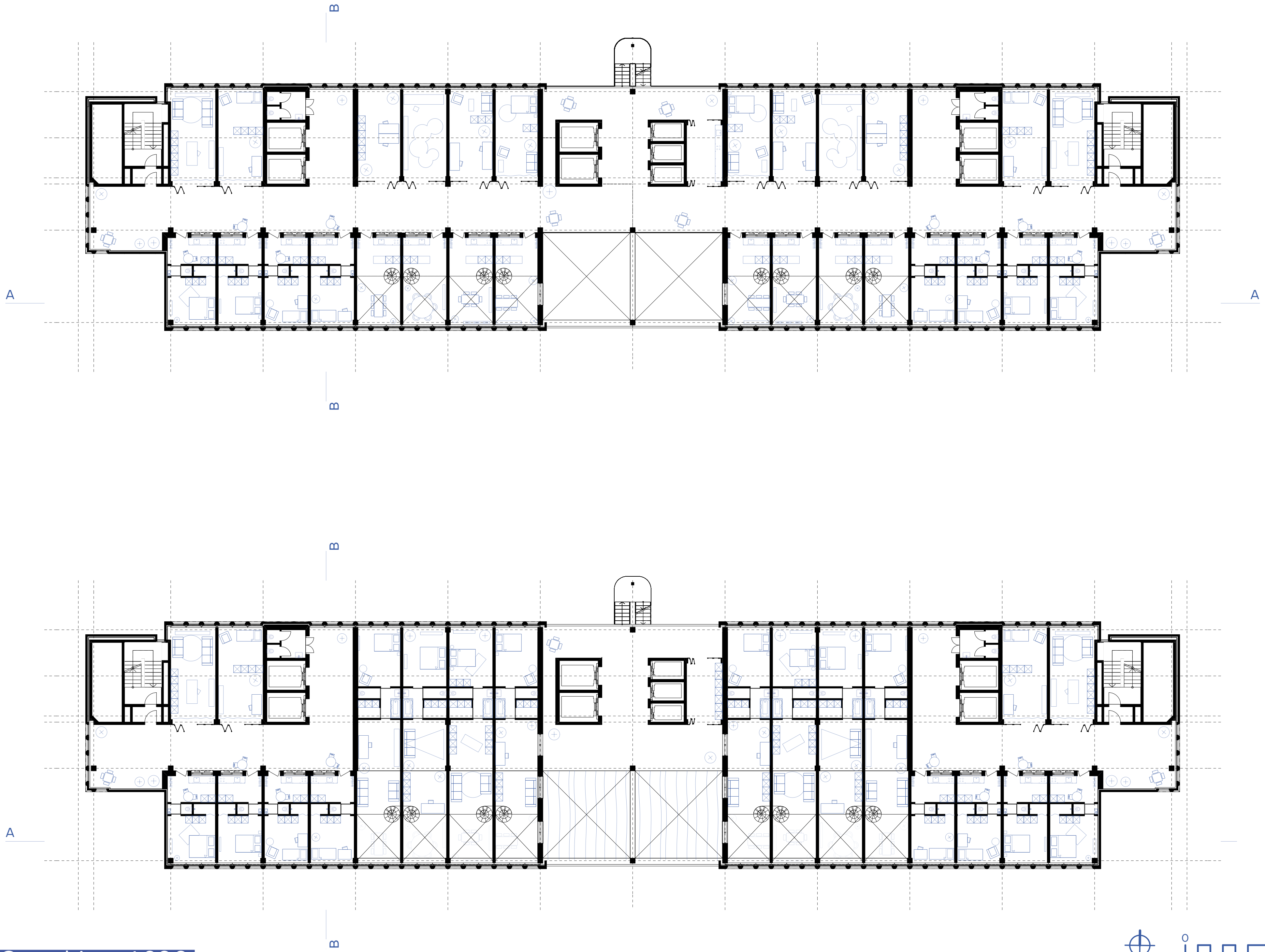
Turm Grundrisse 1:200
