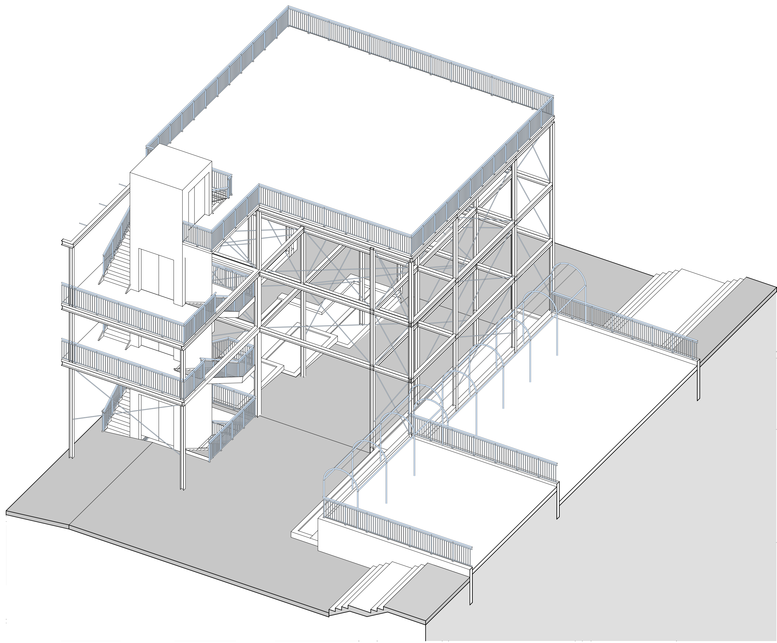
Axonometrie Aussichtsplattform
