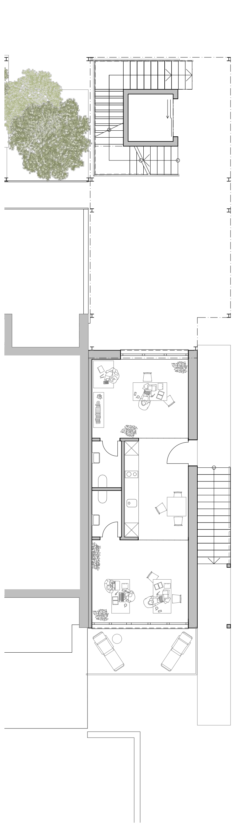
Erdgeschoss, Abstellräume mit Erschließung | Mst. 1:100
