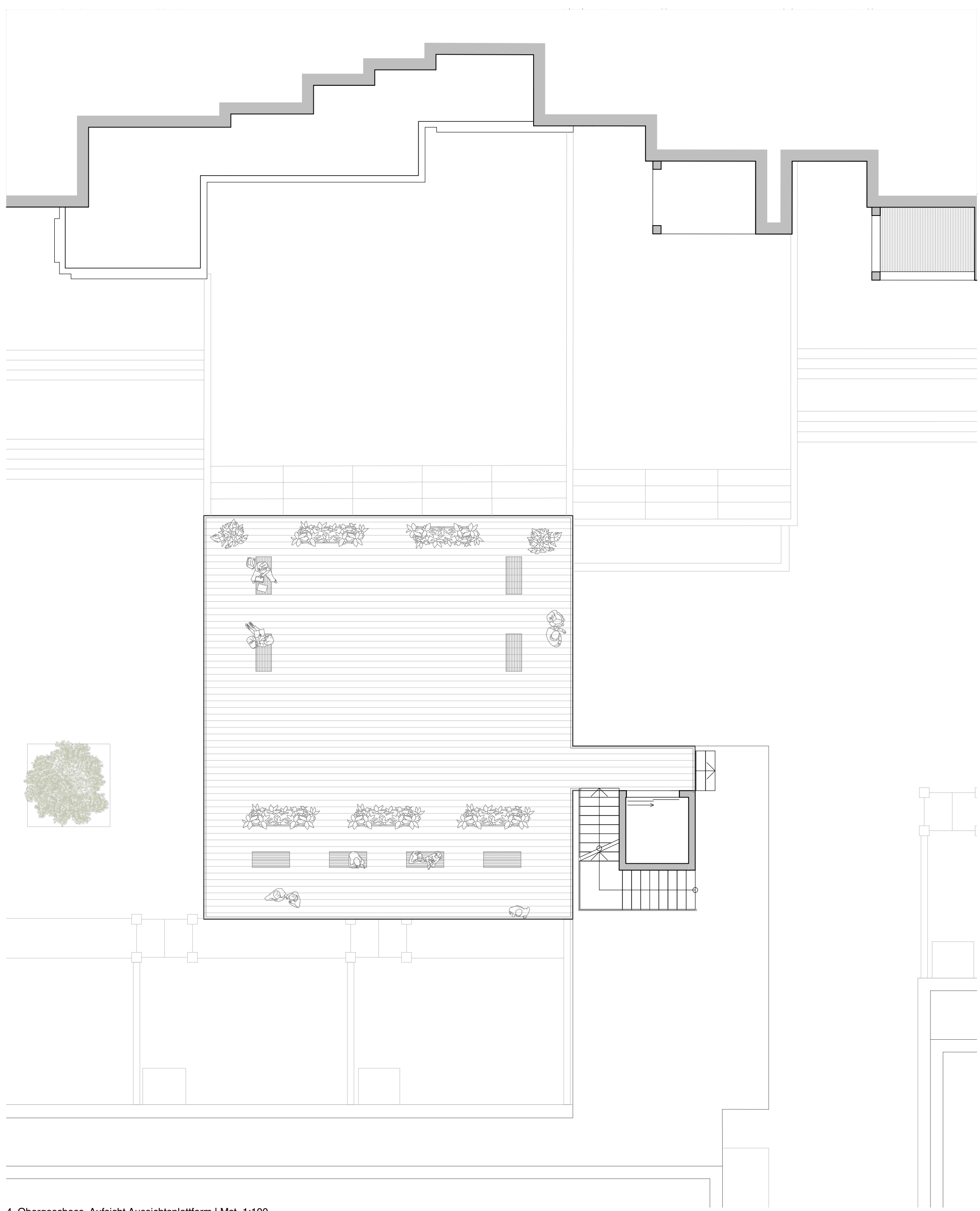
4. Obergeschoss, Aufsicht Aussichtsplattform | Mst. 1:100
