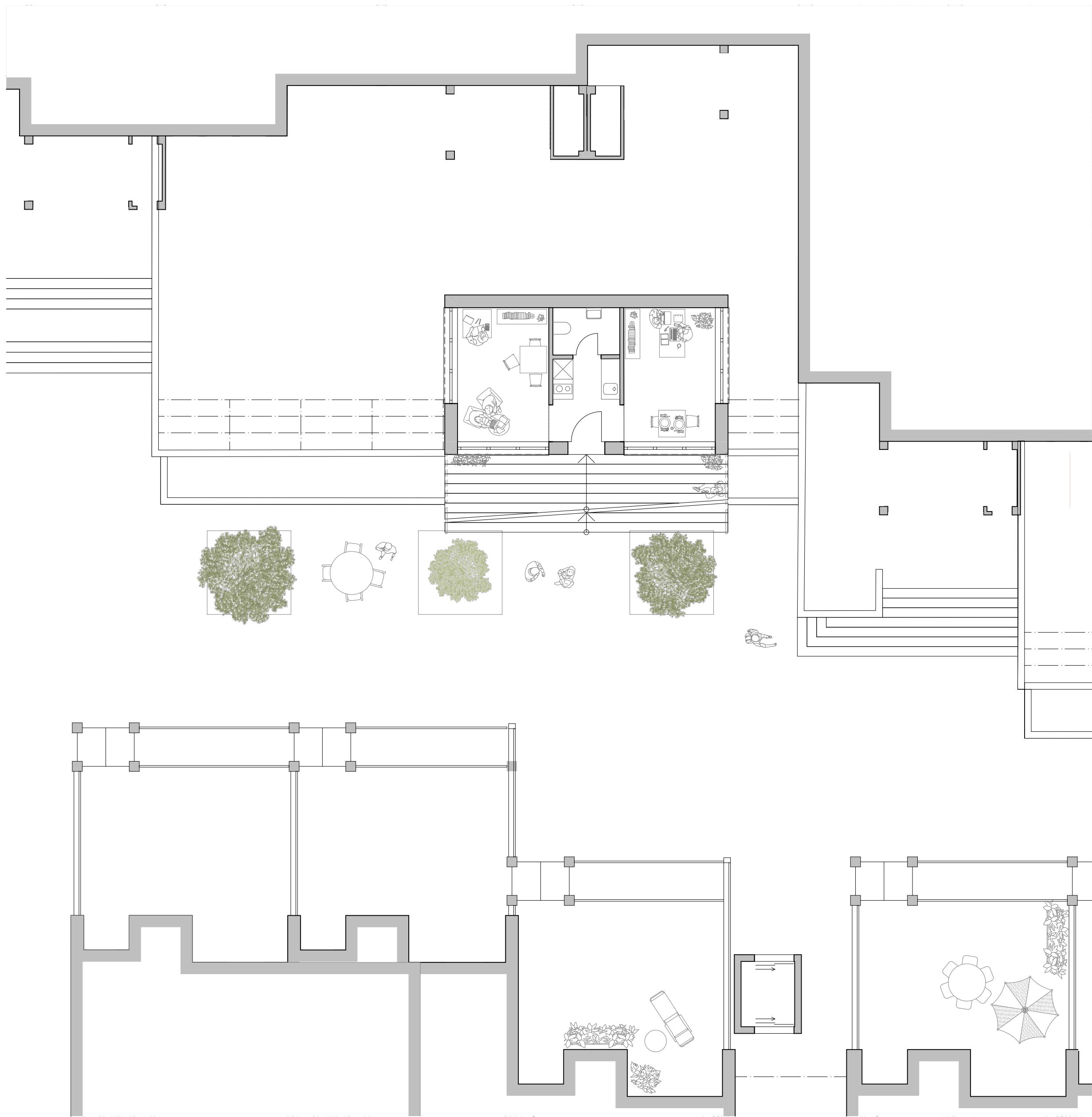
Erdgeschoss, Aulienräume mit Aussenraum | Mst. 1:100
