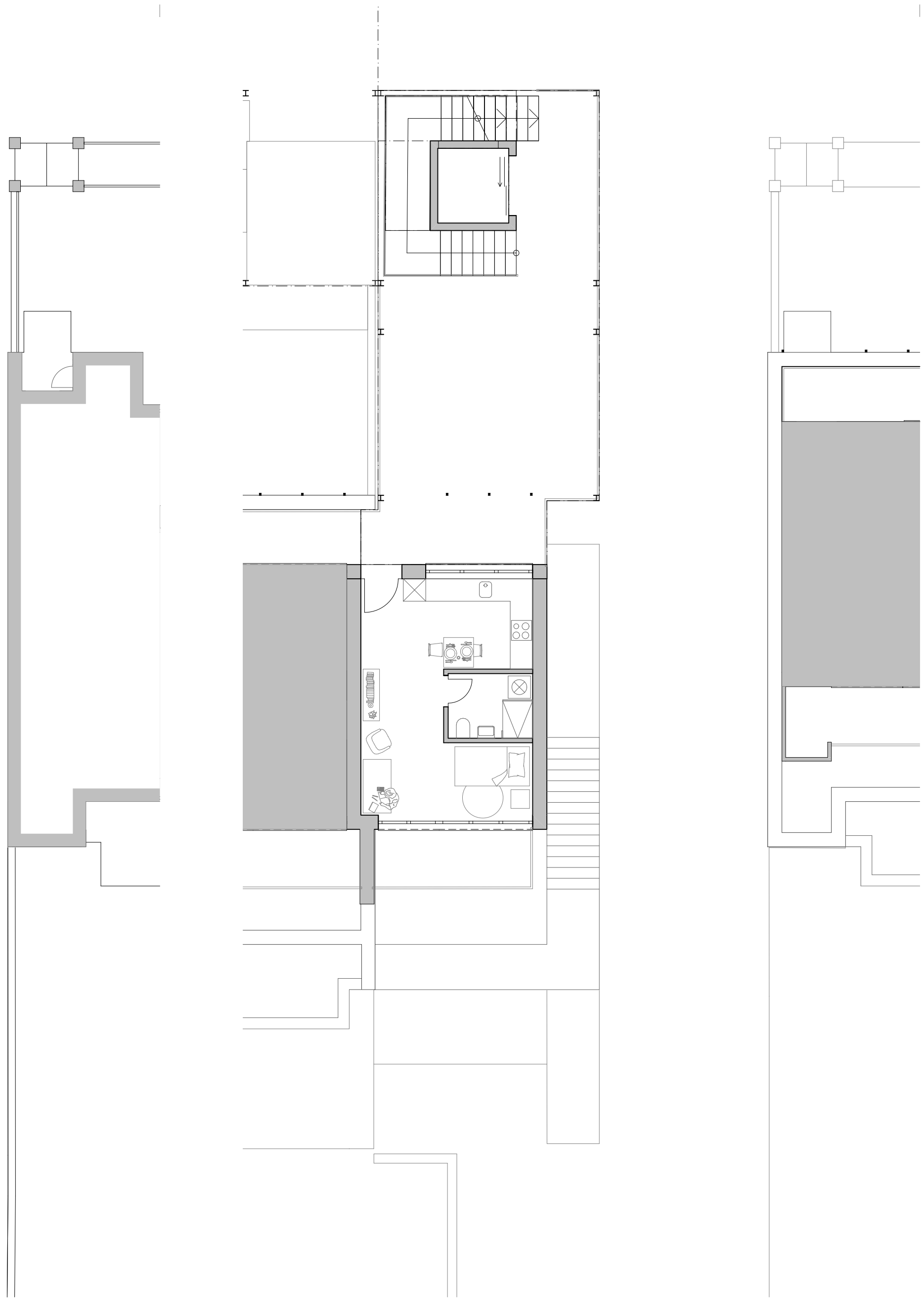
Obergeschoss 2, Kleinwohnung | Mst. 1:100
