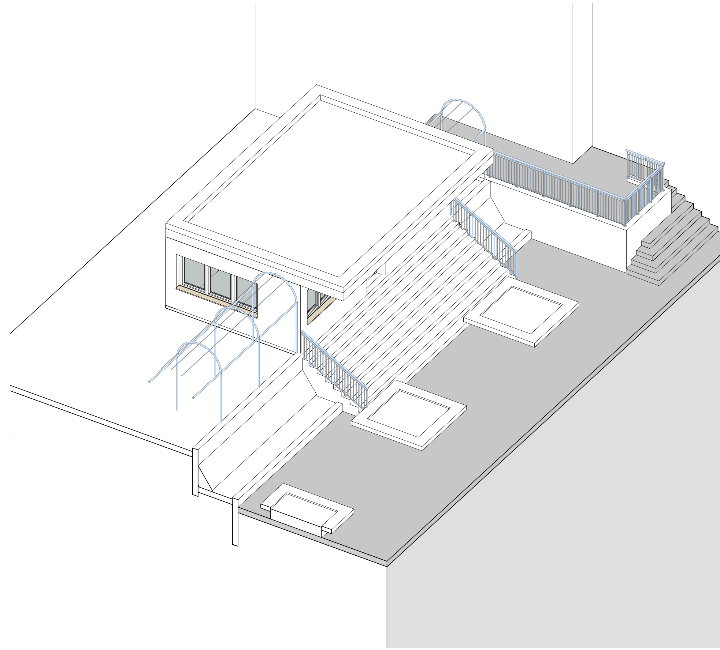
Axonomie Plauderecke
