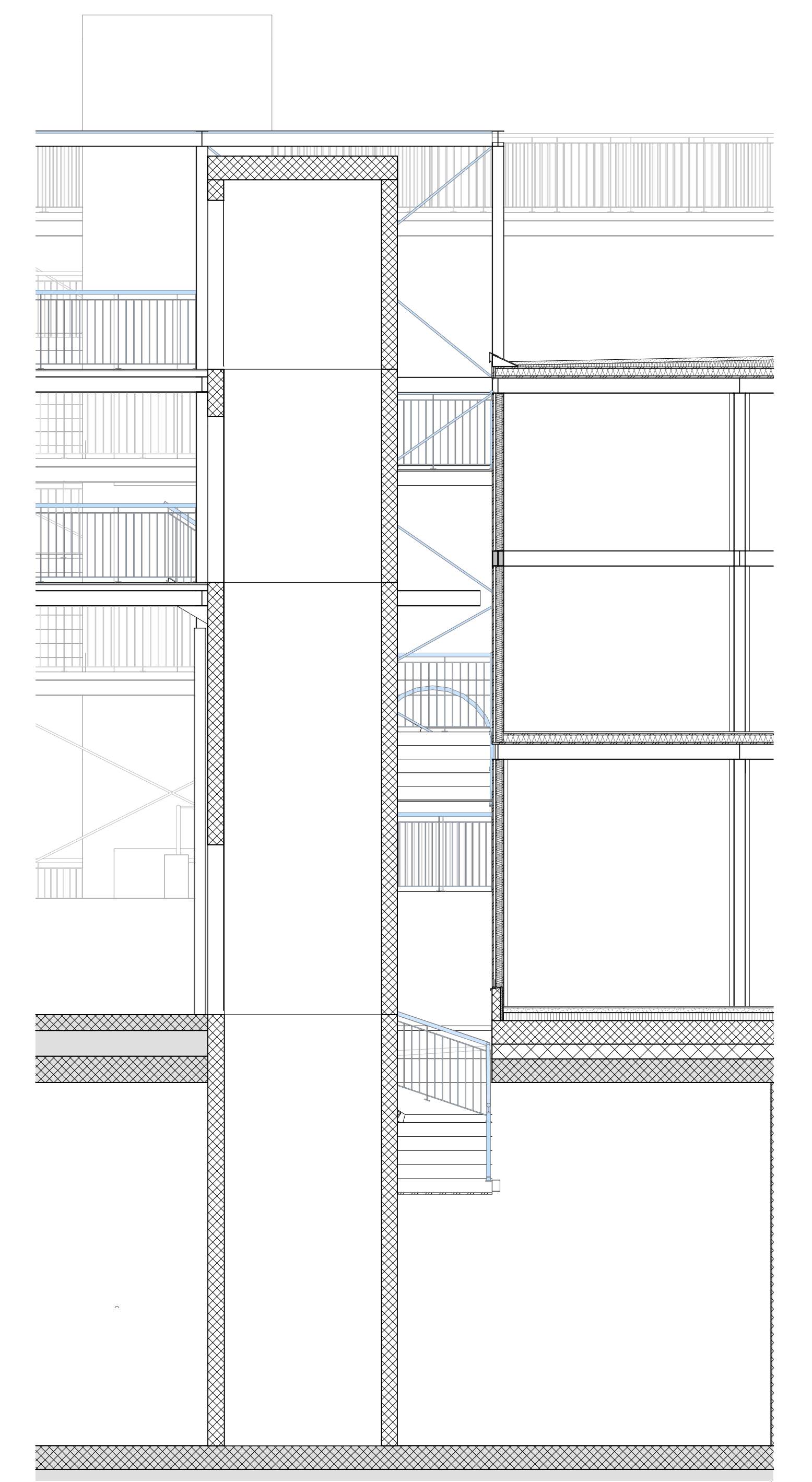
Schnitt Erschliessung und Spielplatzbau | Mst. 1:50
