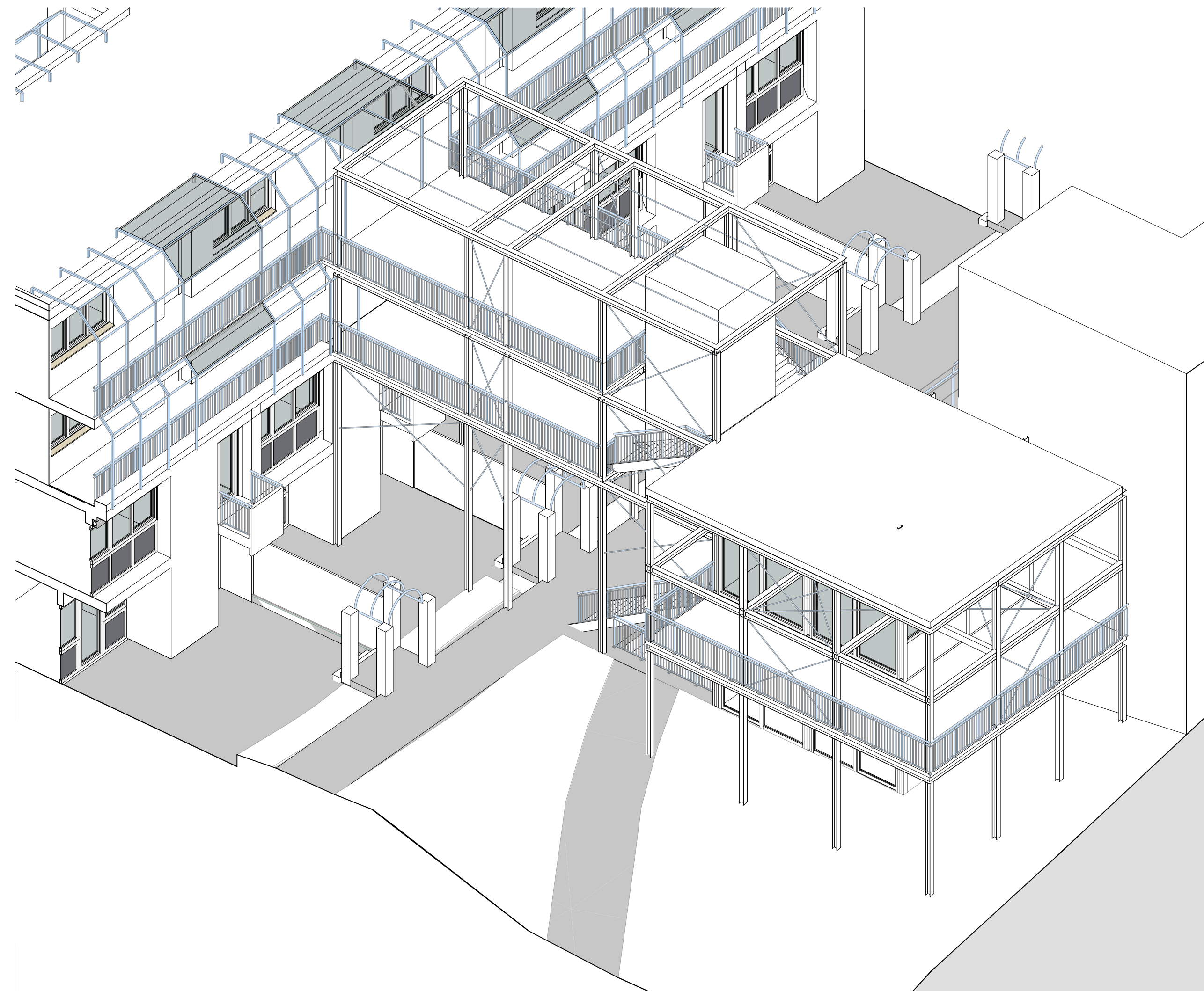
Axonometrie Spielplatz
