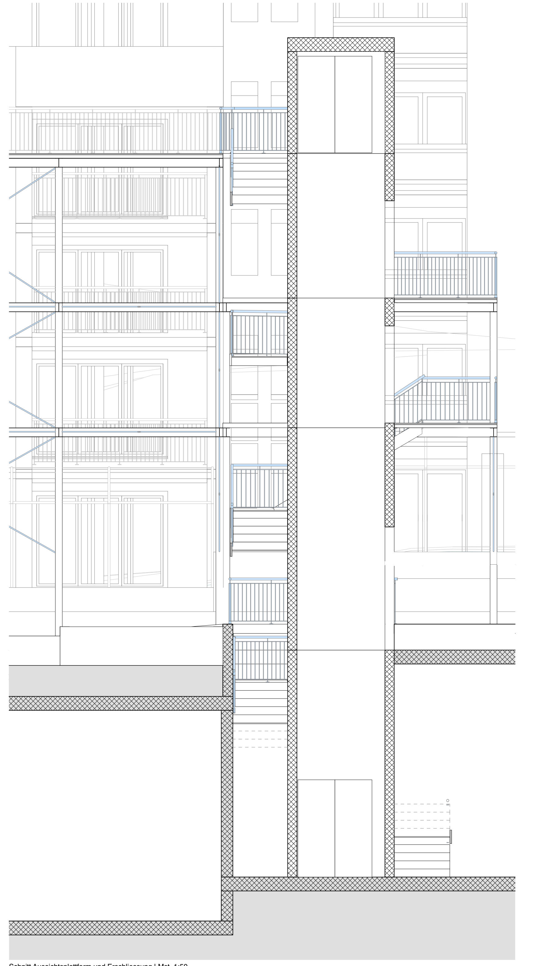
Schnitt Aussichtsplattform und Erschliessung | Mst. 1:50
