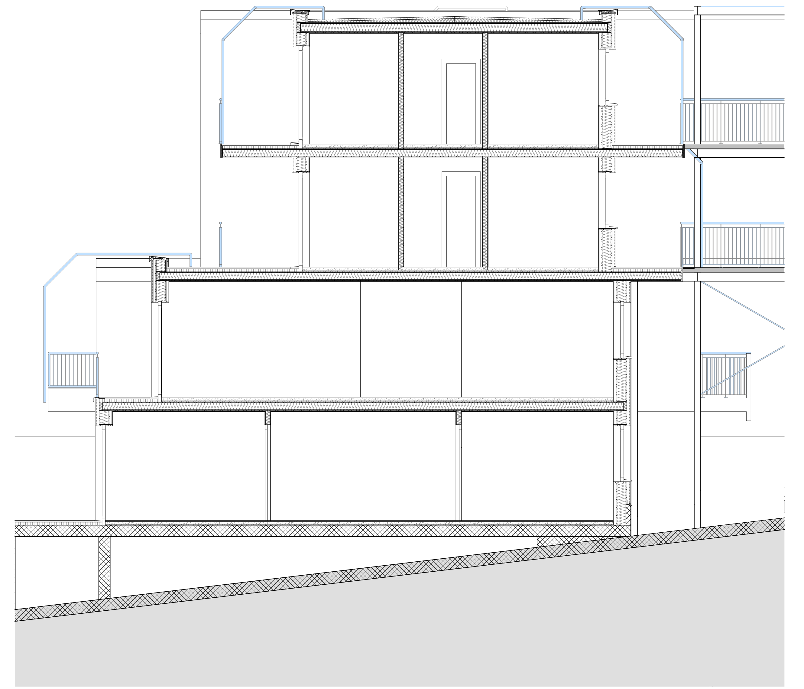
Schnitt Abstell- und Wohnraum | Mst. 1:50
