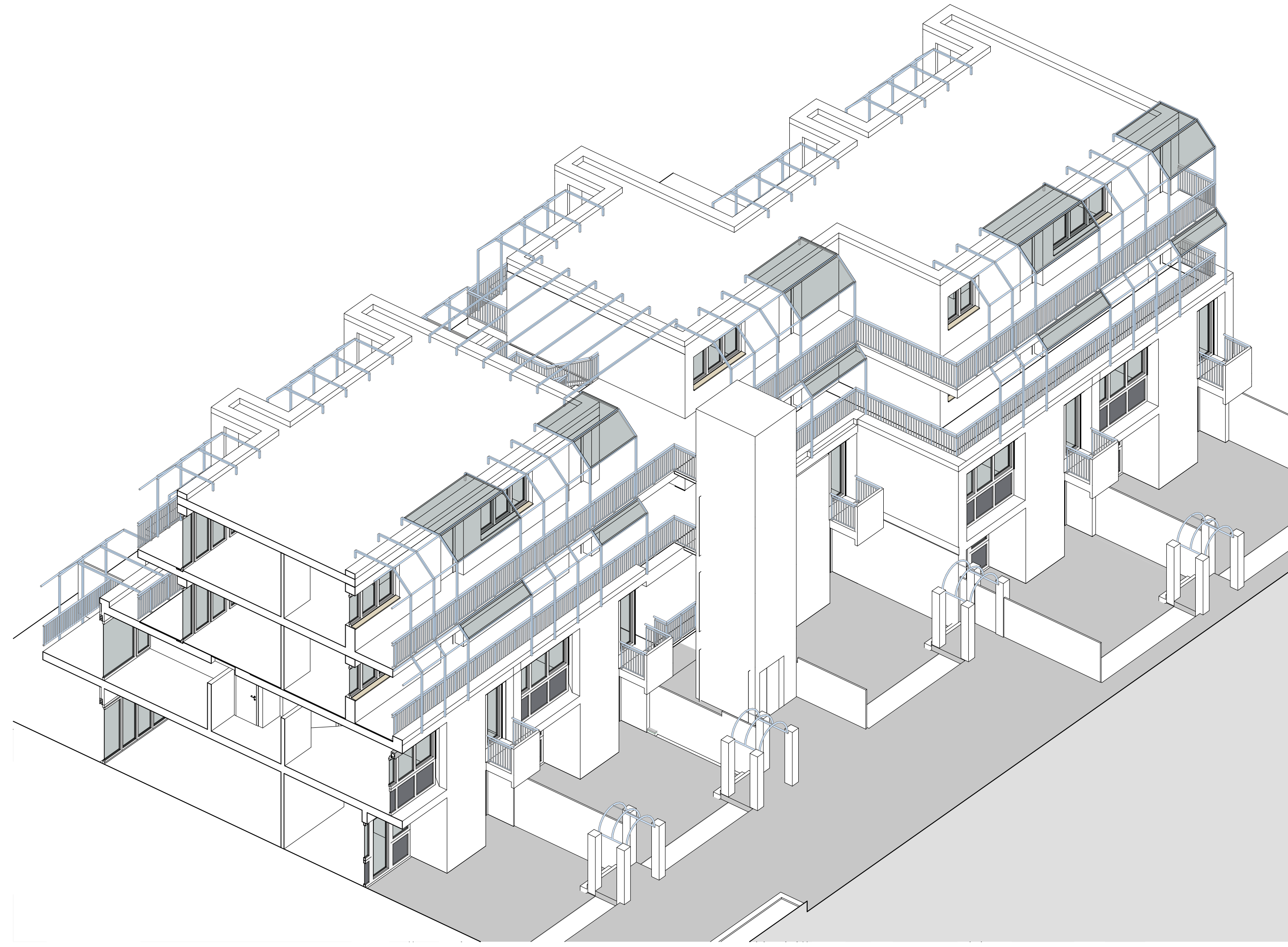
Axonometrie Aufstockung
