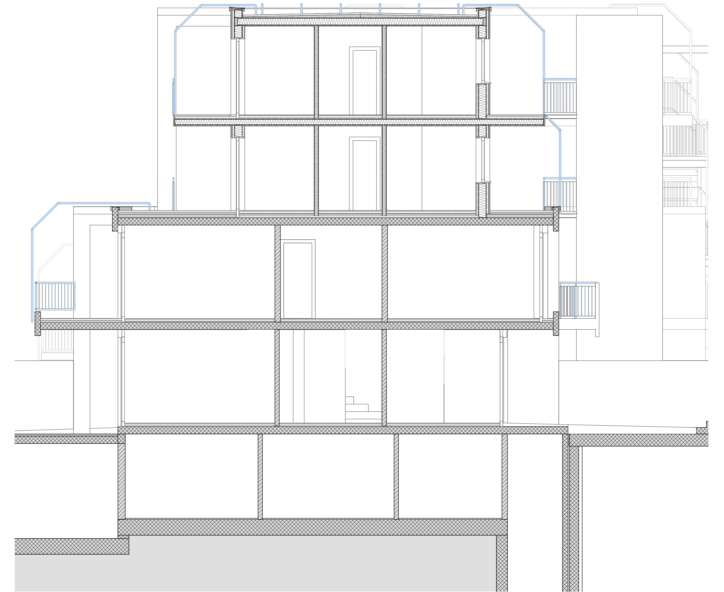
Schnitt Bestand mit Aufstockung | Mst. 1:50
