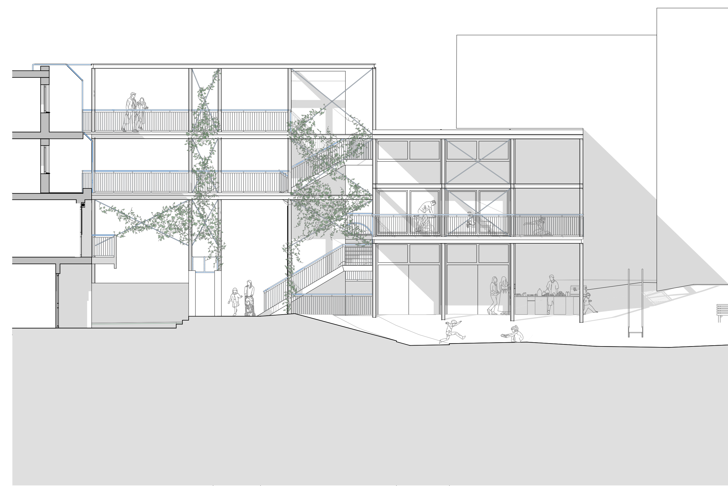
Ansicht Spielplatzbau | Mst. 1:100
