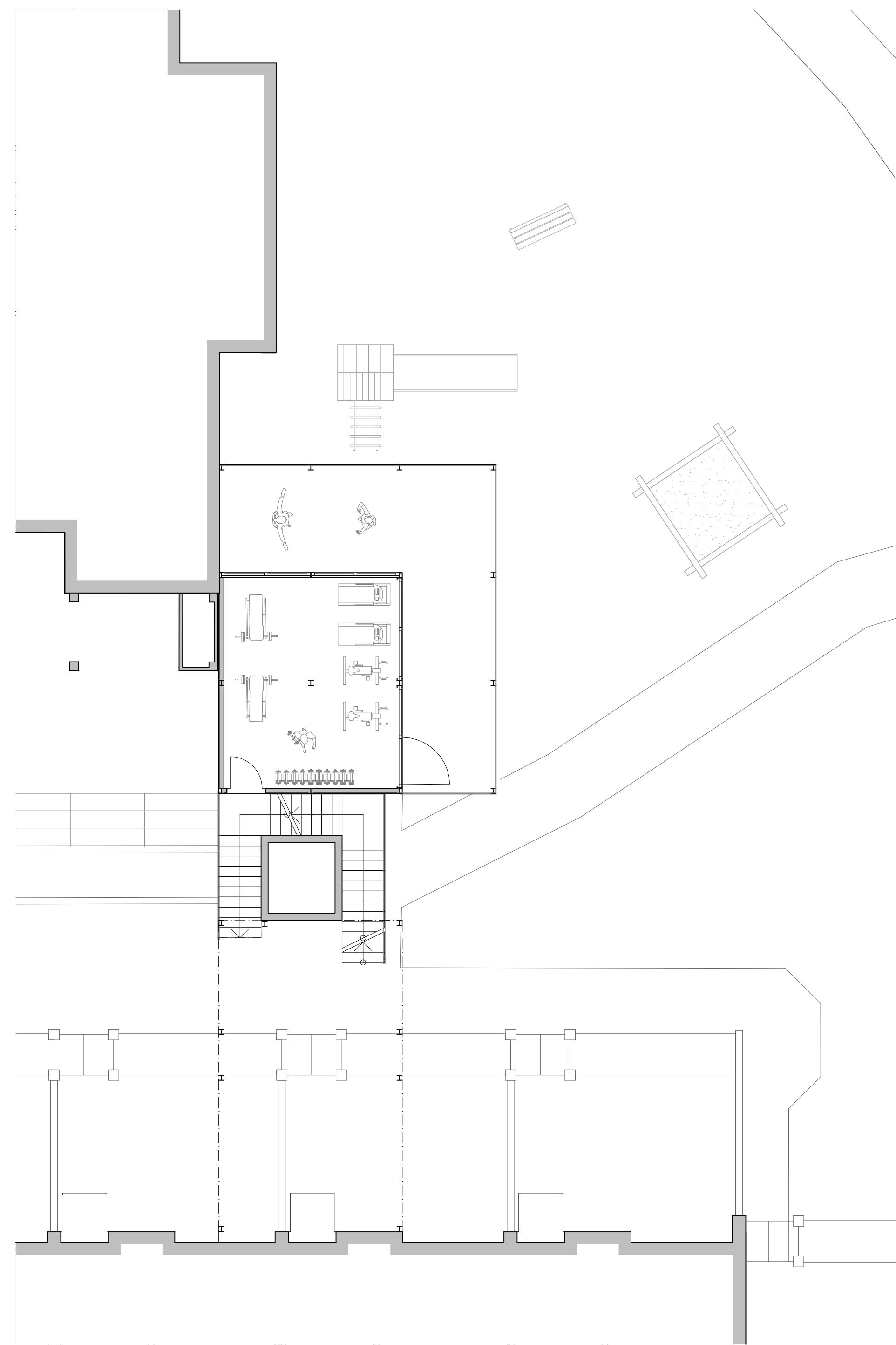
Obergeschoss 1, Sportraum mit Erschliessung | Mst. 1:100
