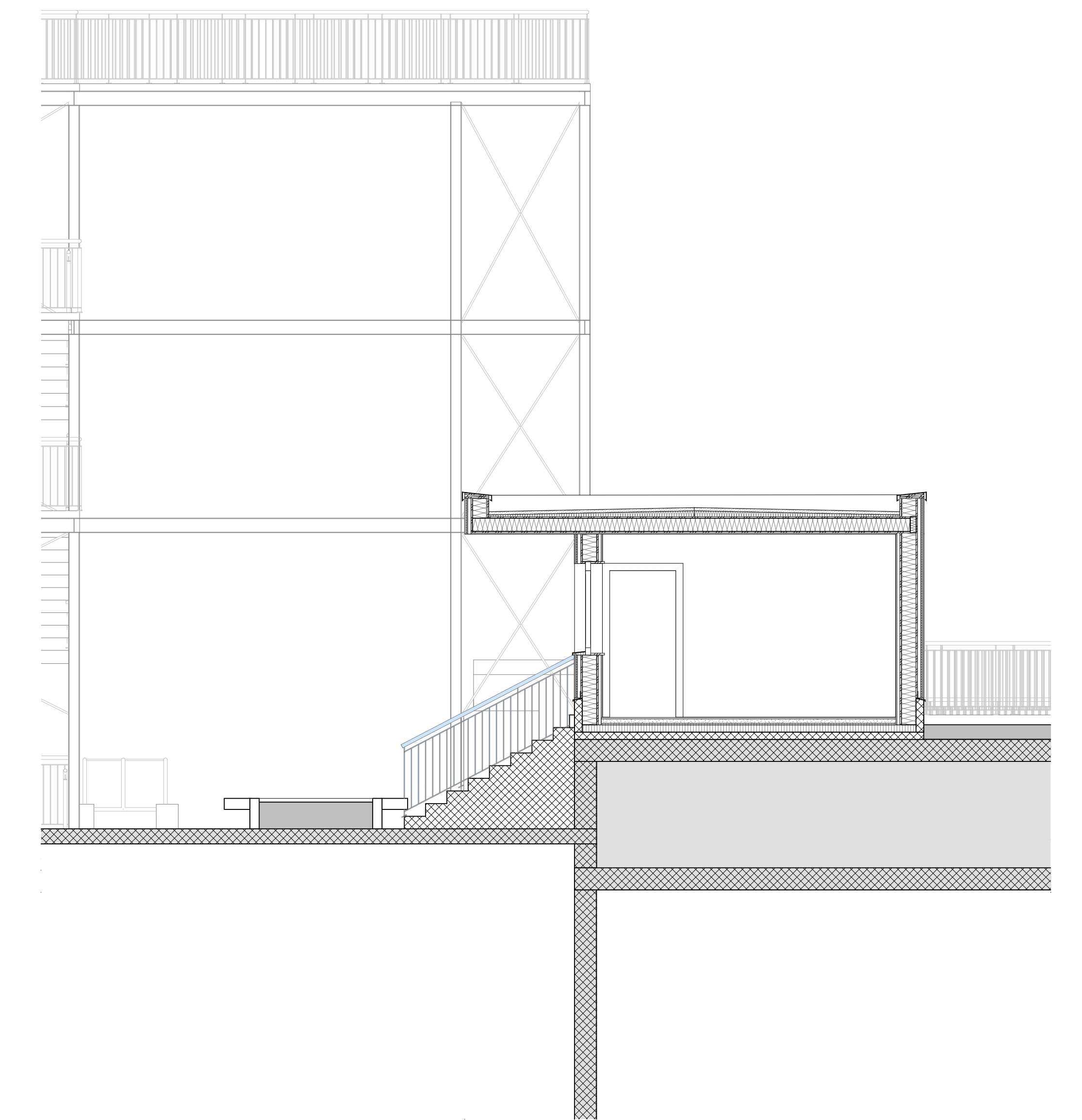
Schnitt Aulienräume | Mst. 1:50
