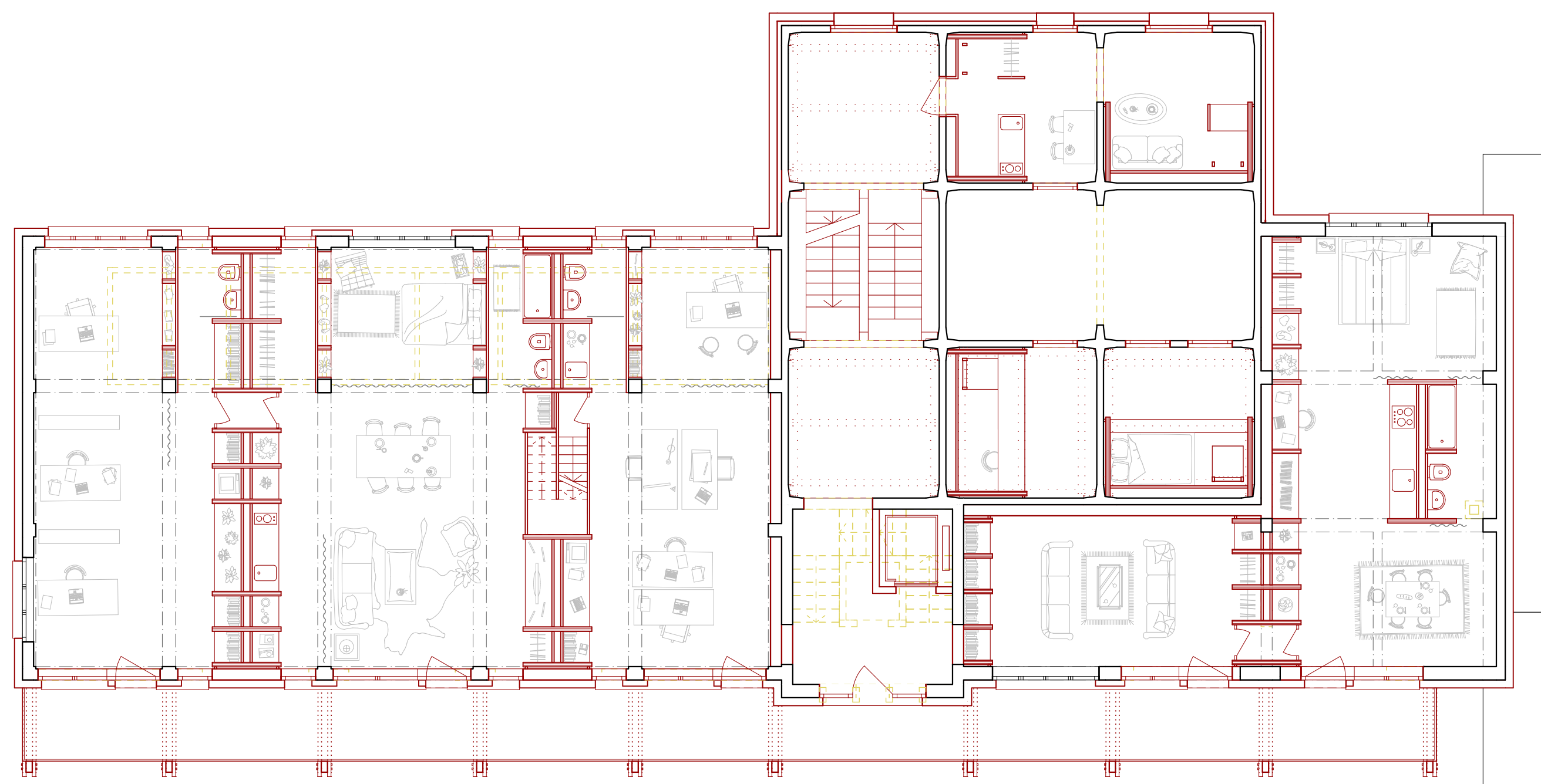
3. Obergeschoss 1:100 2m
