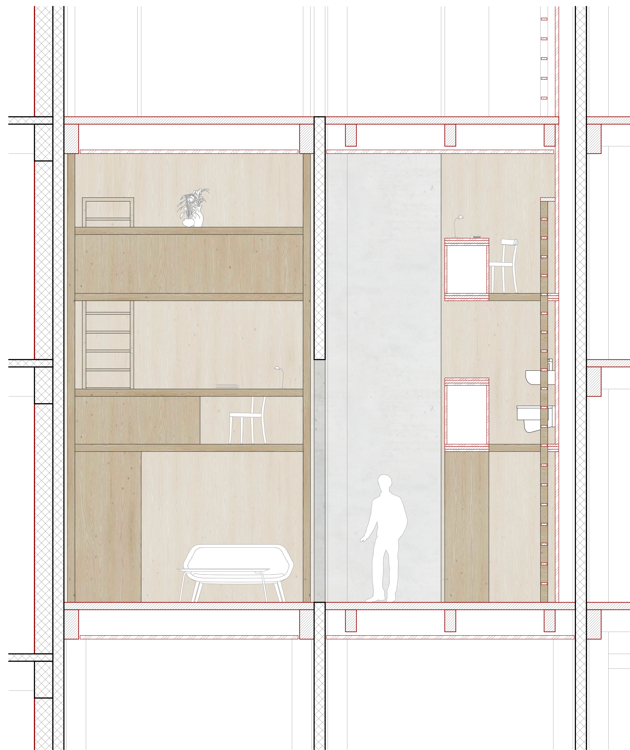
Detailschnitt vertikales Wohnen — 60cm —
