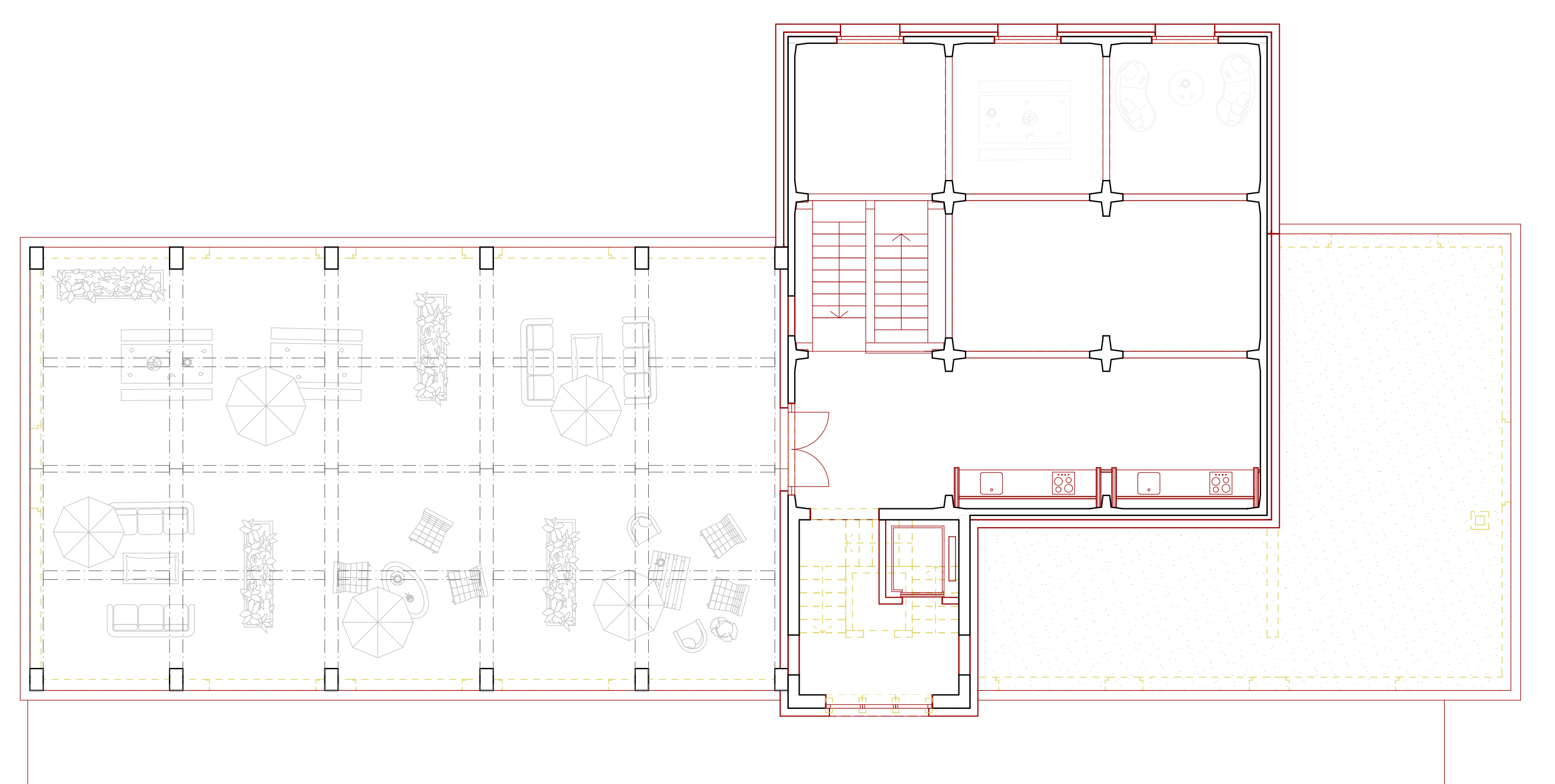
Dachgeschoss 1:100 2m
