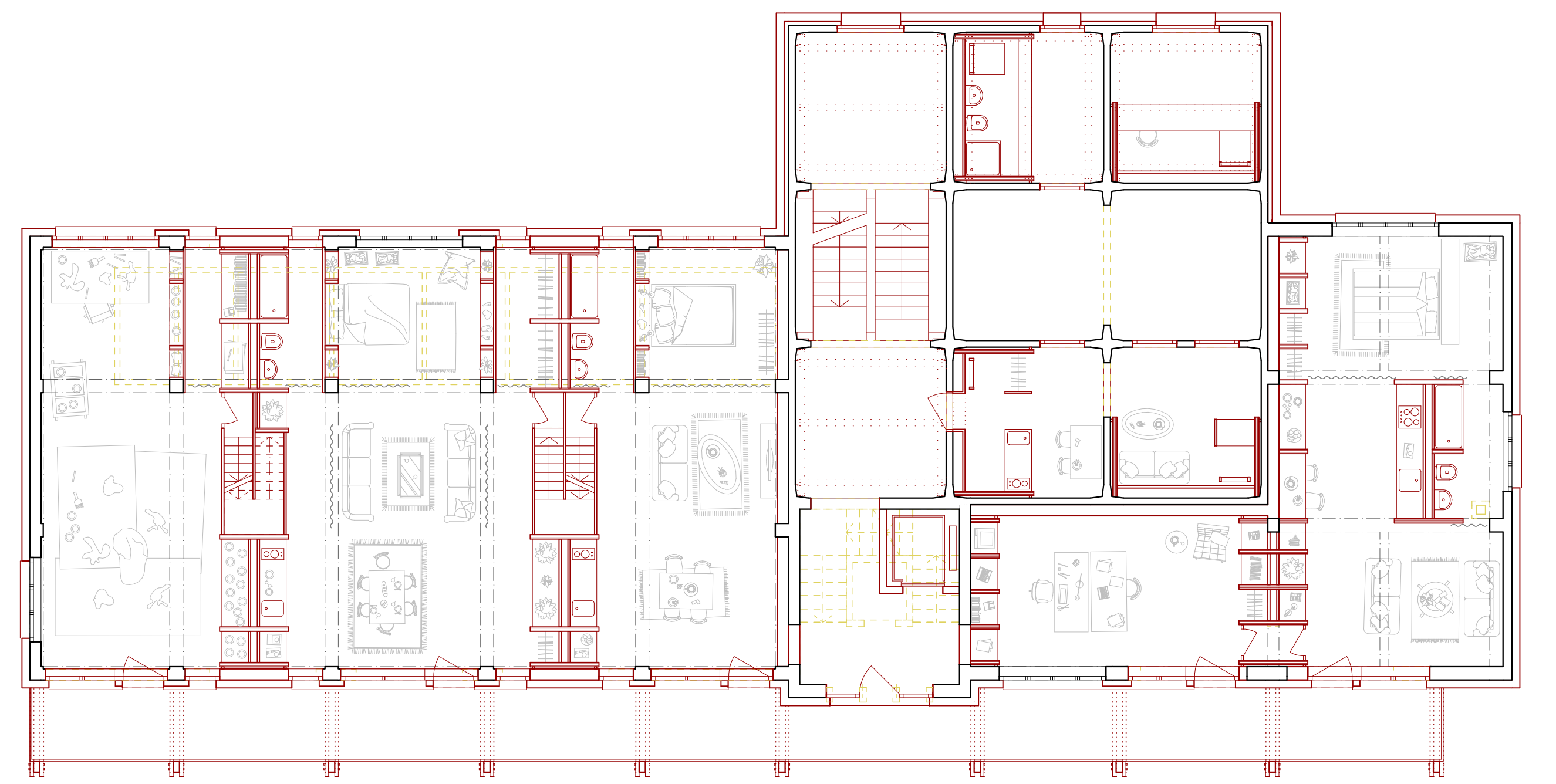
4. Obergeschoss 1:100 2m
