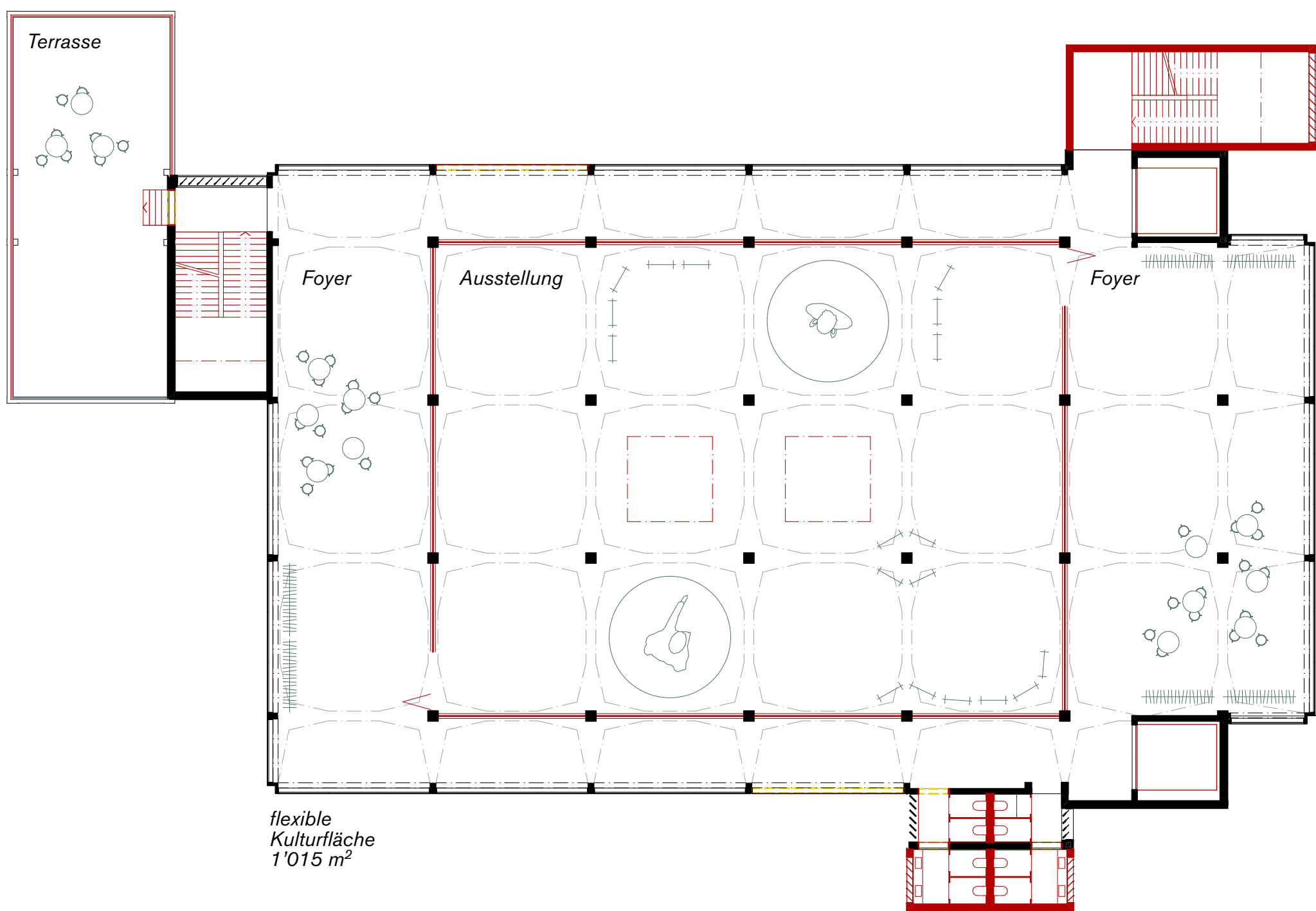
2. Obergeschoss 1:200
