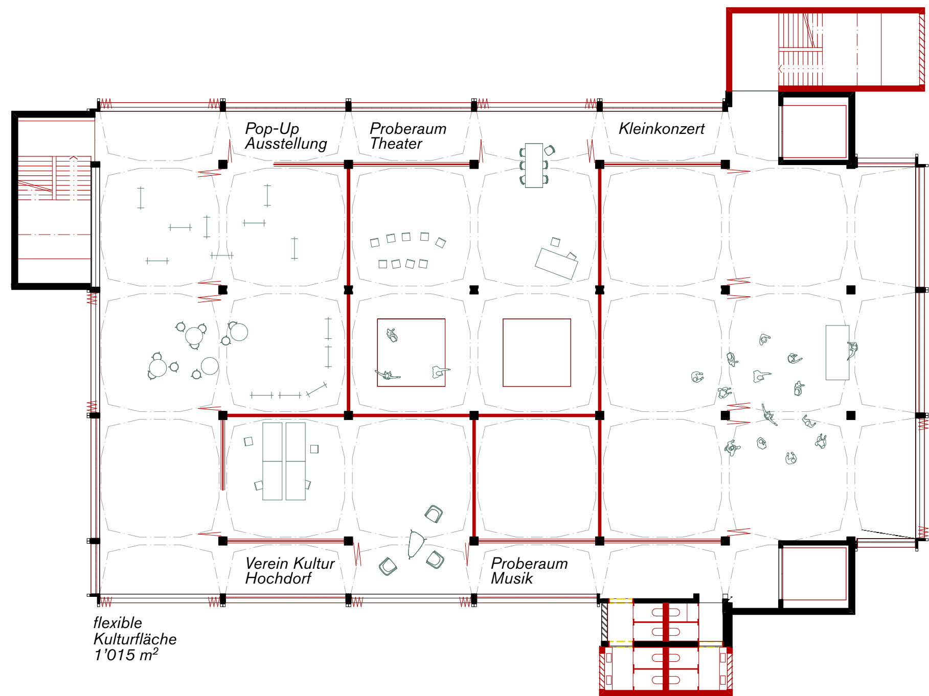
3. Obergeschoss 1:200
