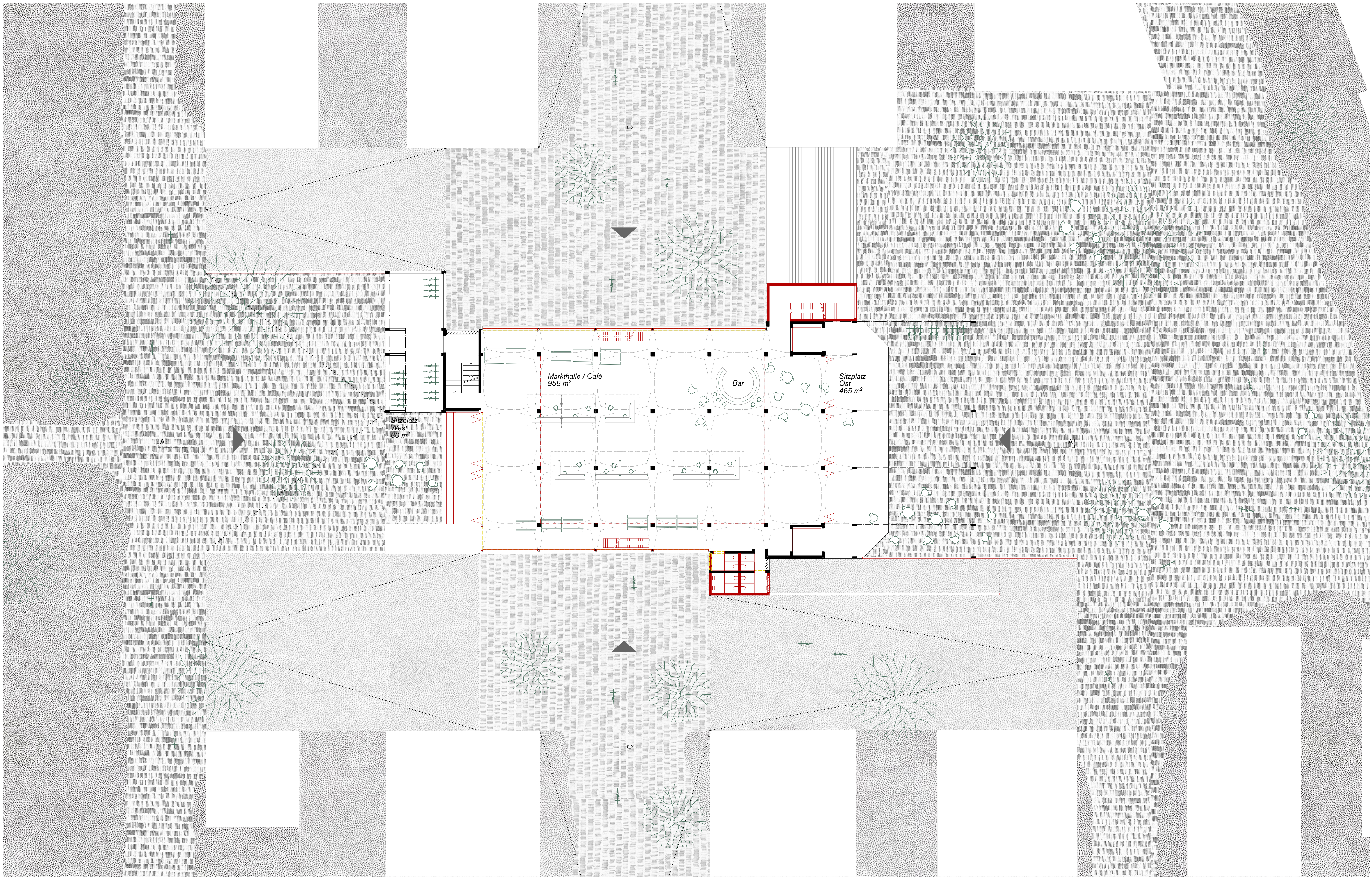
Erdgeschoss mit Umgebung 1:200
