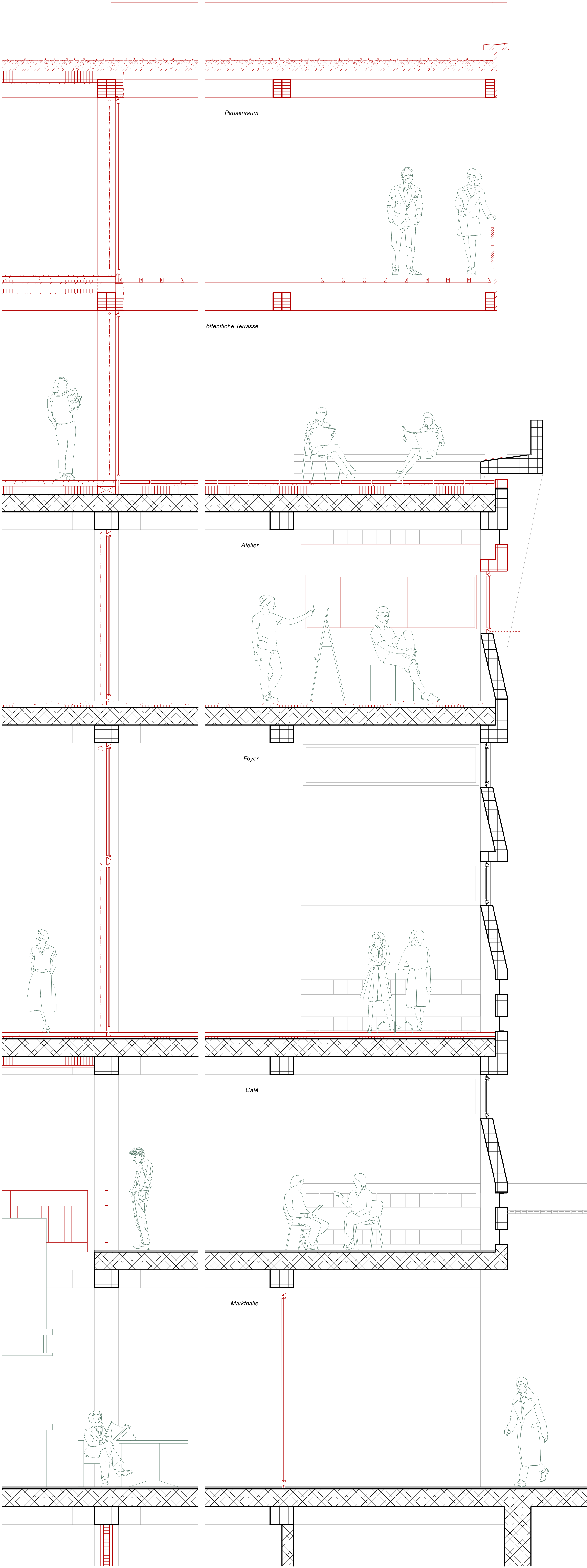
Fassadenschnitt 1:25
