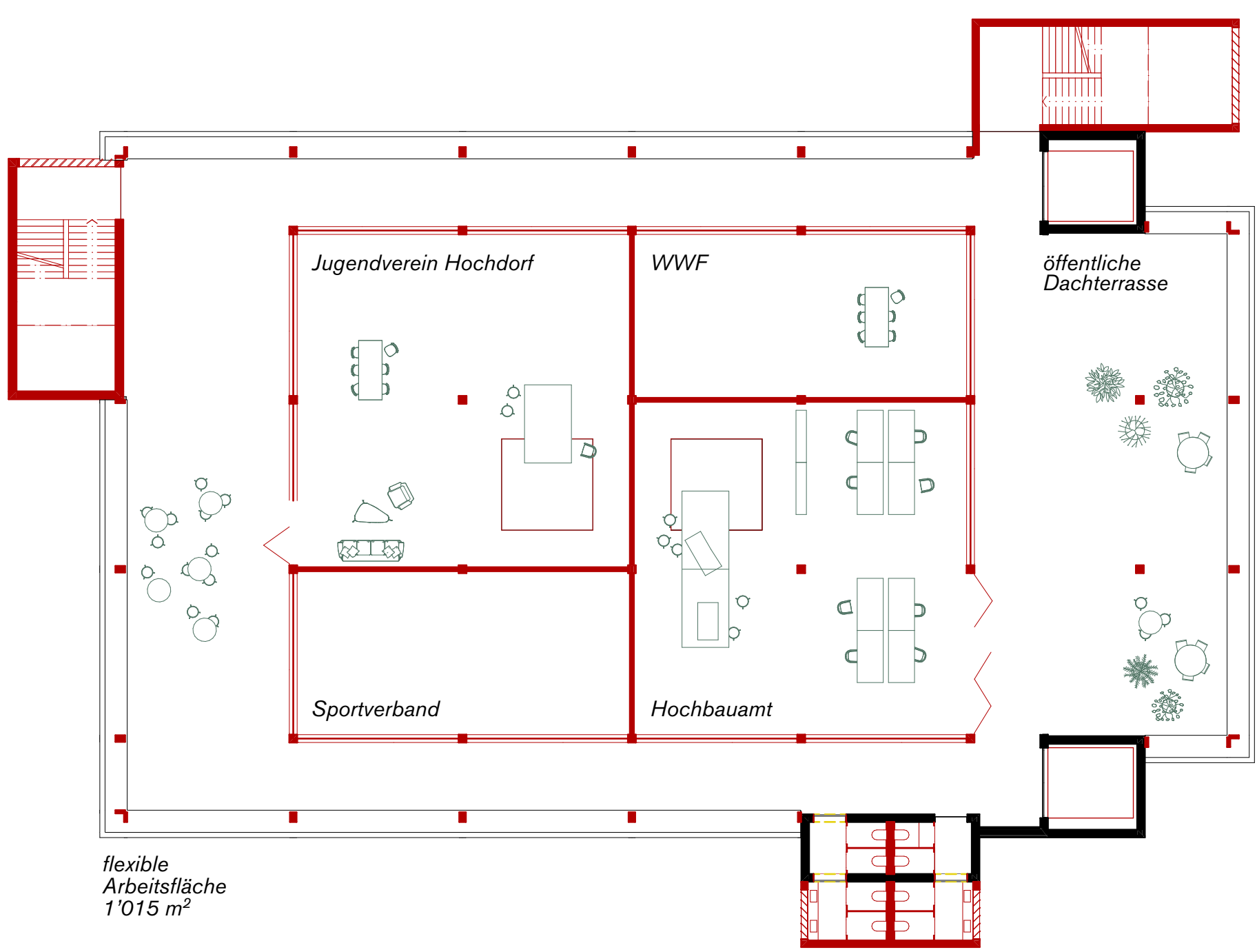
4. Obergeschoss 1:200
