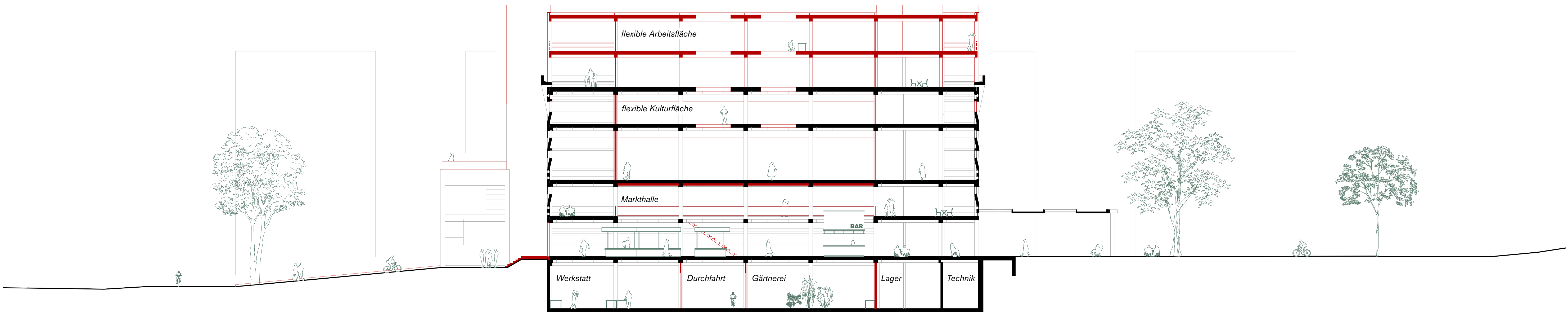
Längsschnitt A 1:200
