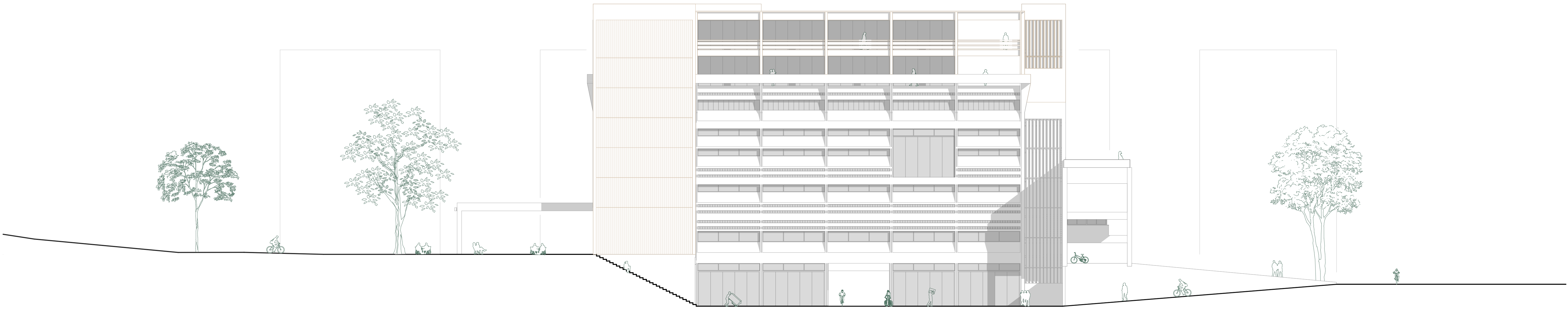
Nordfassade 1:200
