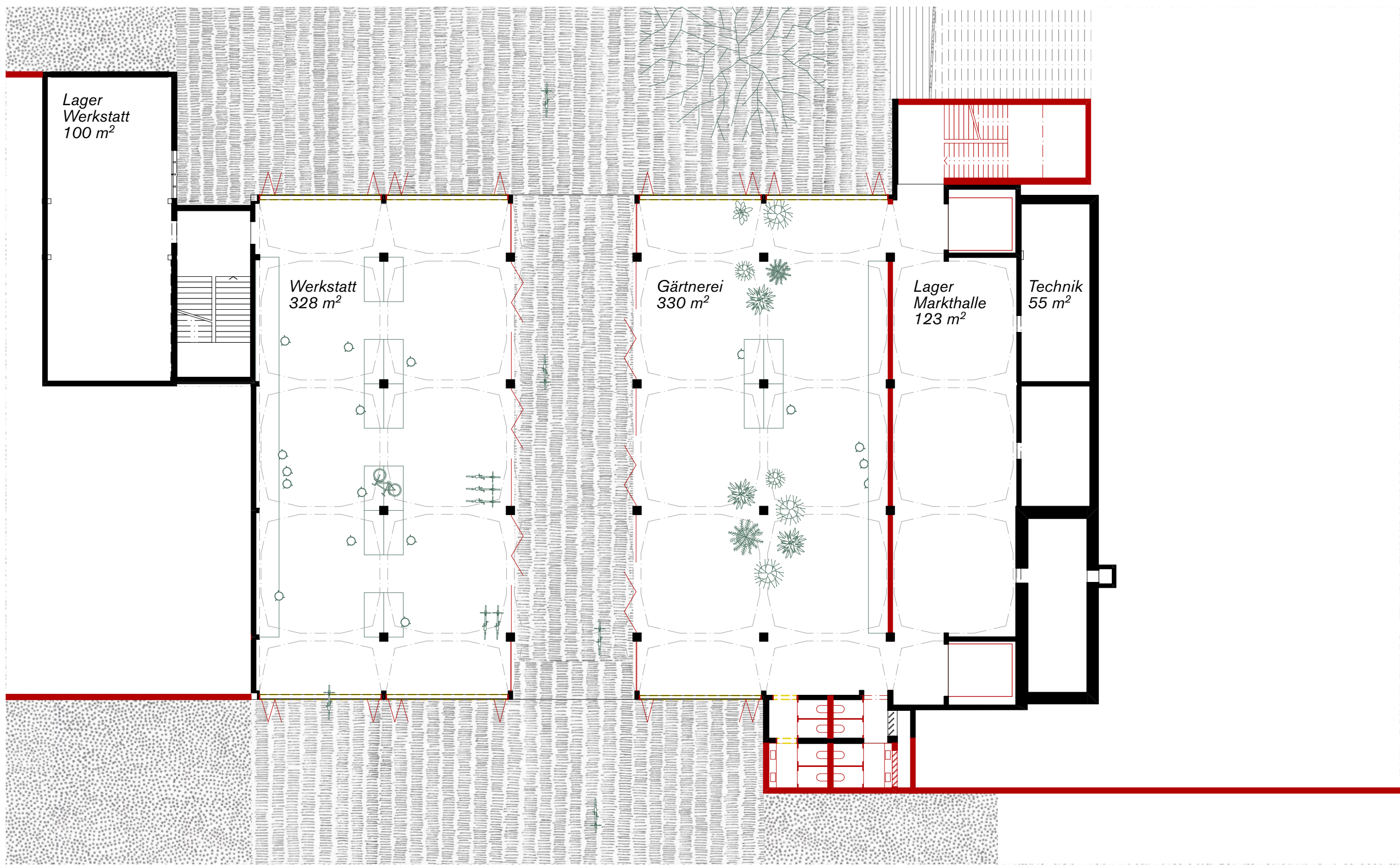
Untergeschoss 1:200
