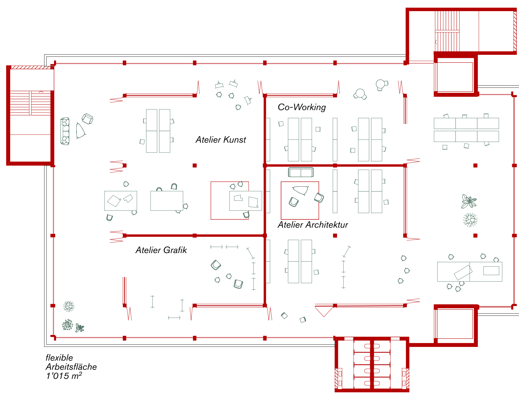
5. Obergeschoss 1:200
