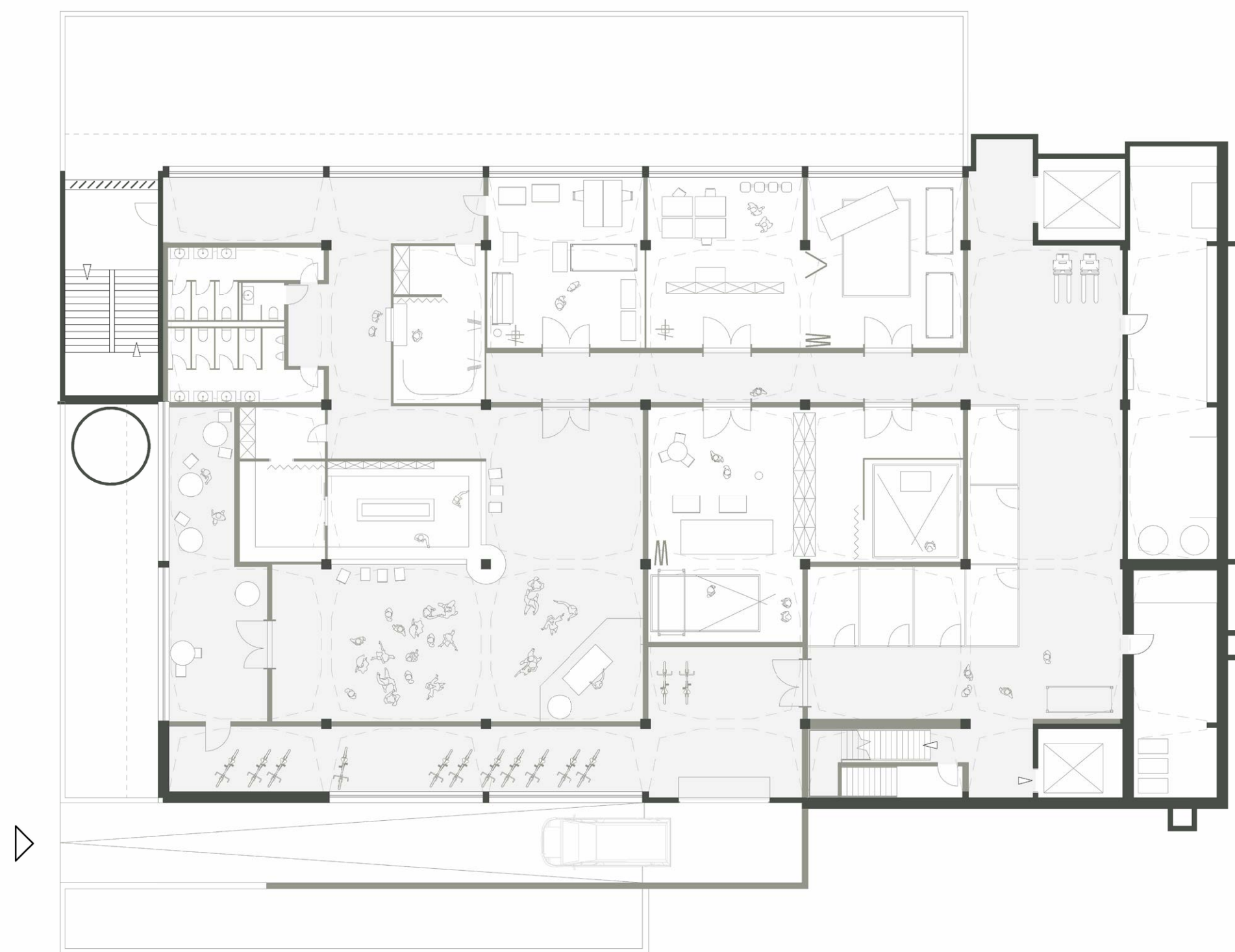
UNTERGESCHOSS
