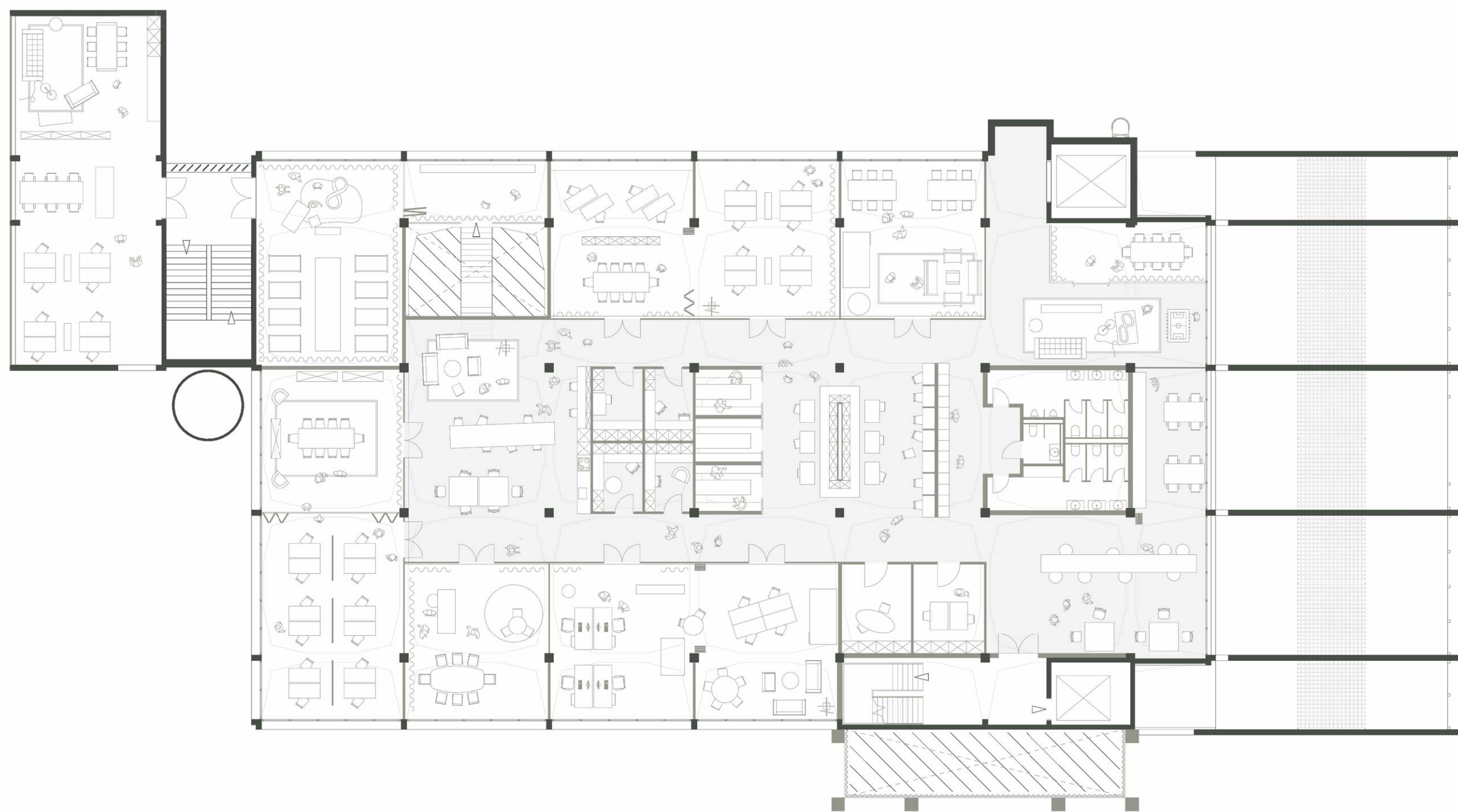
1. OBERGESCHOSS
