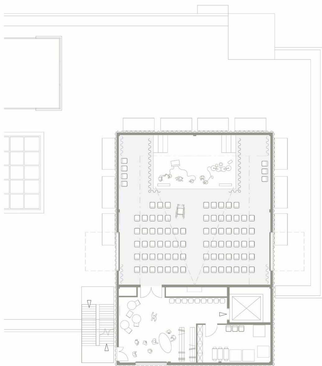
TURMGESCHOSS II
