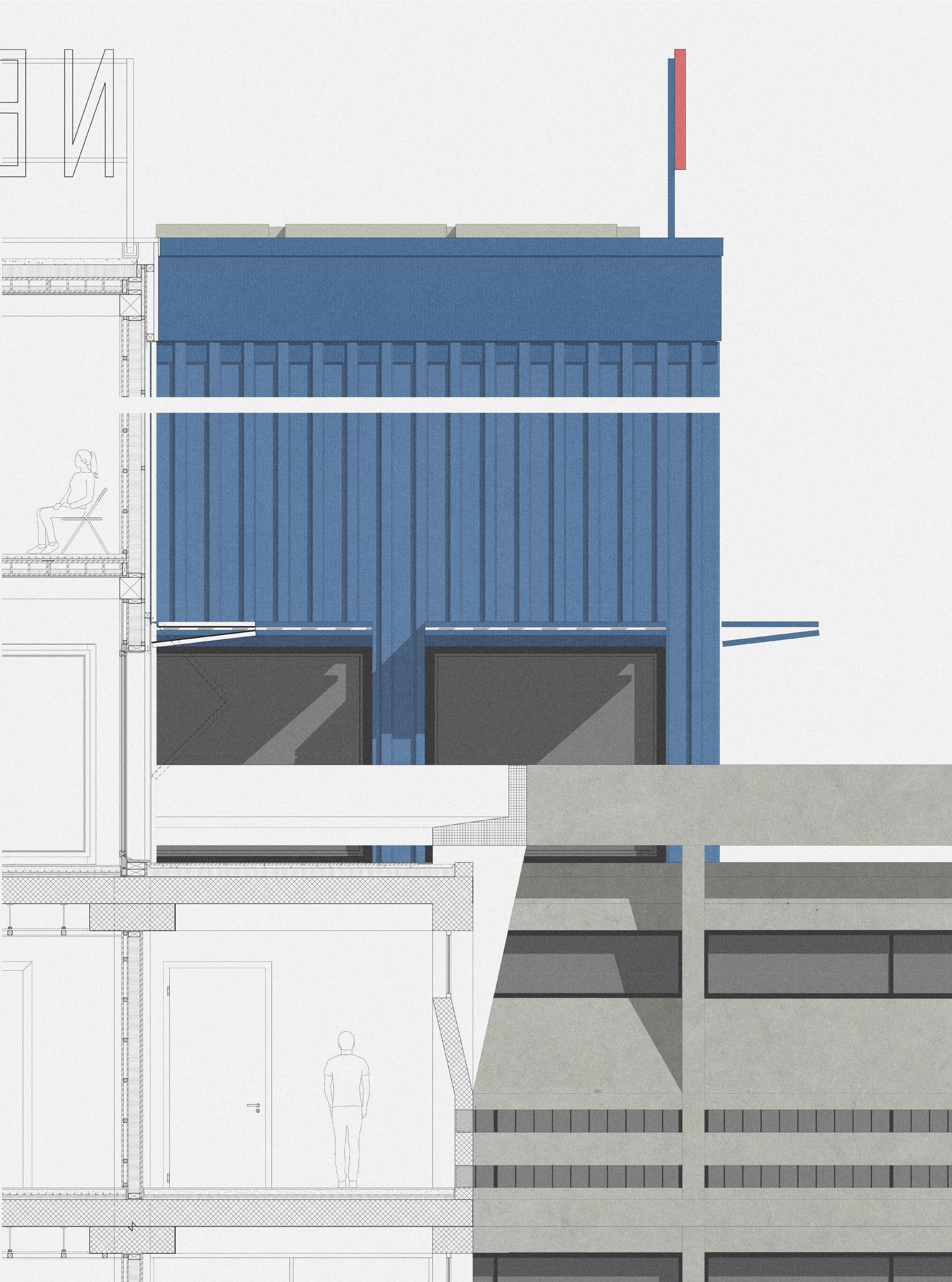
fassadenschnitt .
