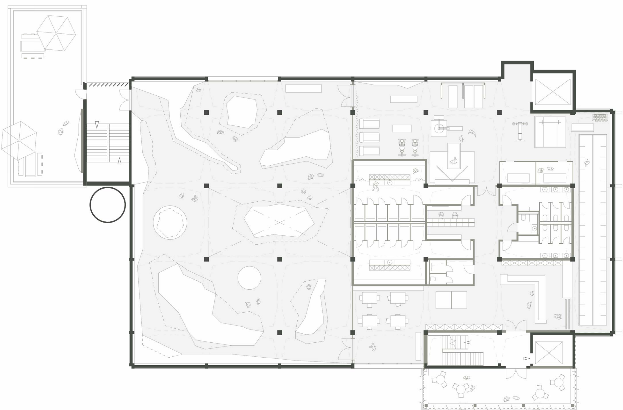
2. OBERGESCHOSS
