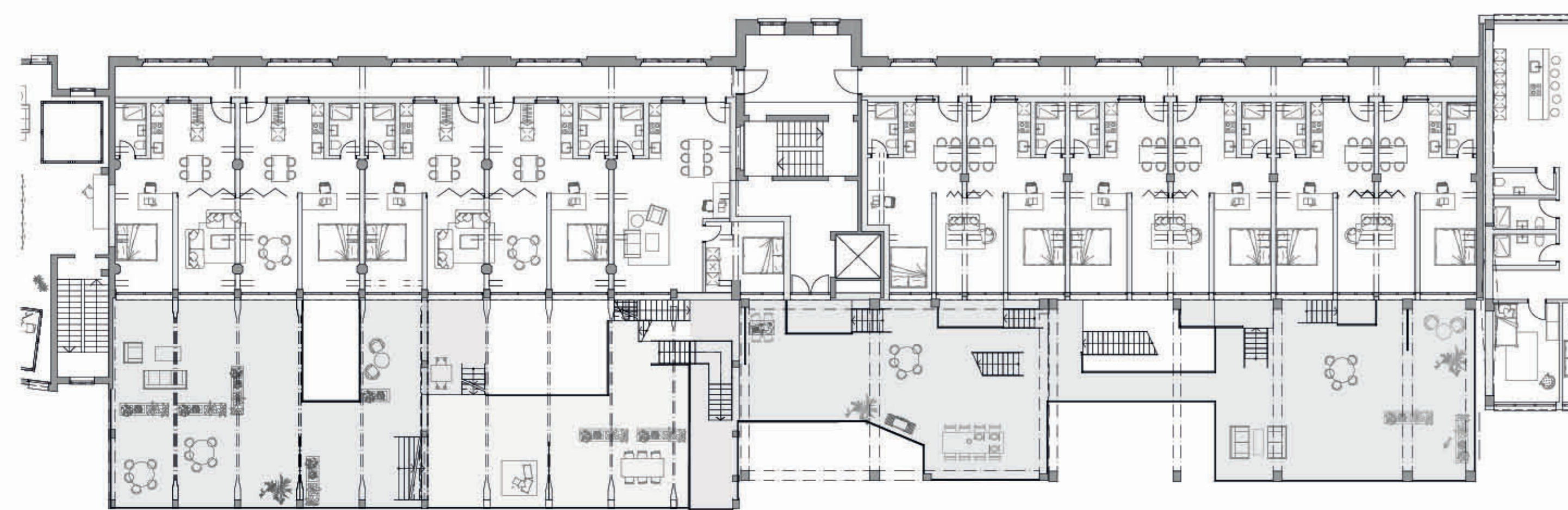
Grundriss 1.Obergeschoss | 1:200
