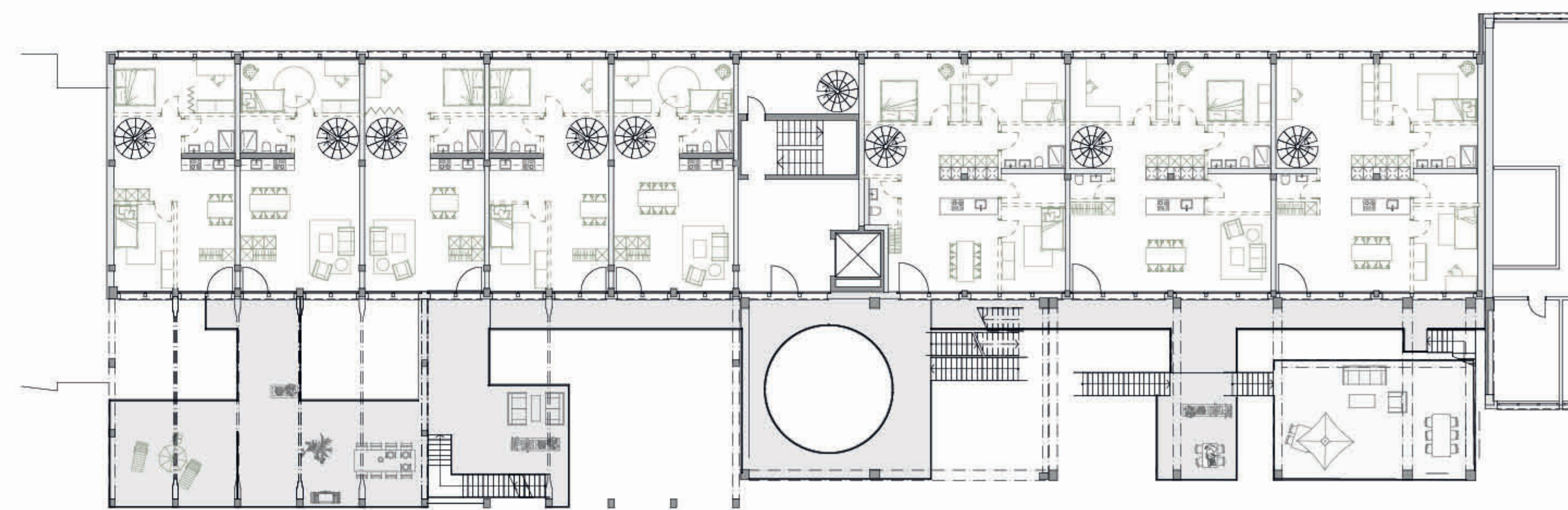
Grundriss 3.Obergeschoss (Aufstockung) | 1:200
