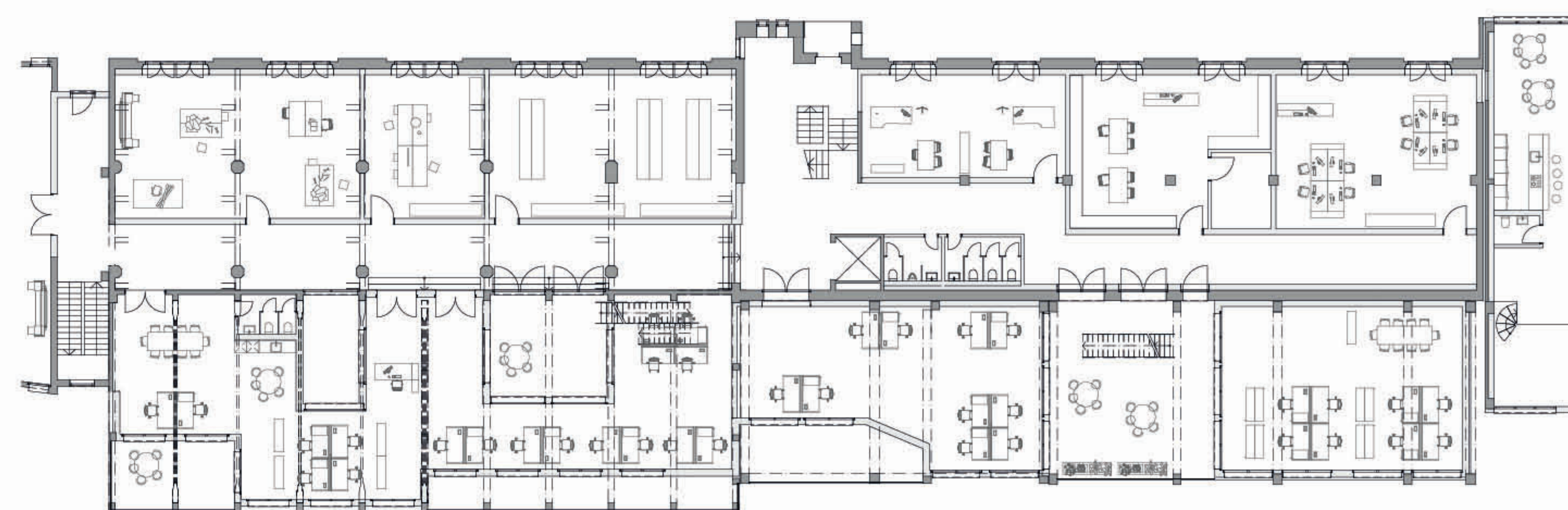
Grundriss Erdgeschoss | 1:200
