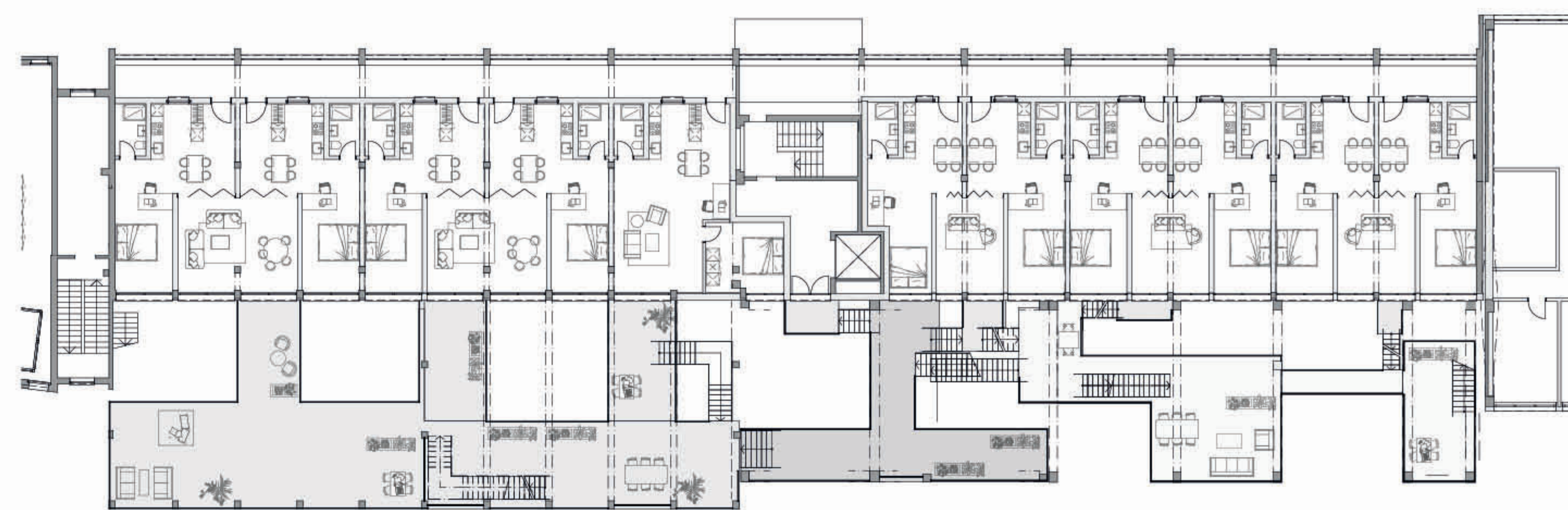
Grundriss 2.Obergeschoss | 1:200
