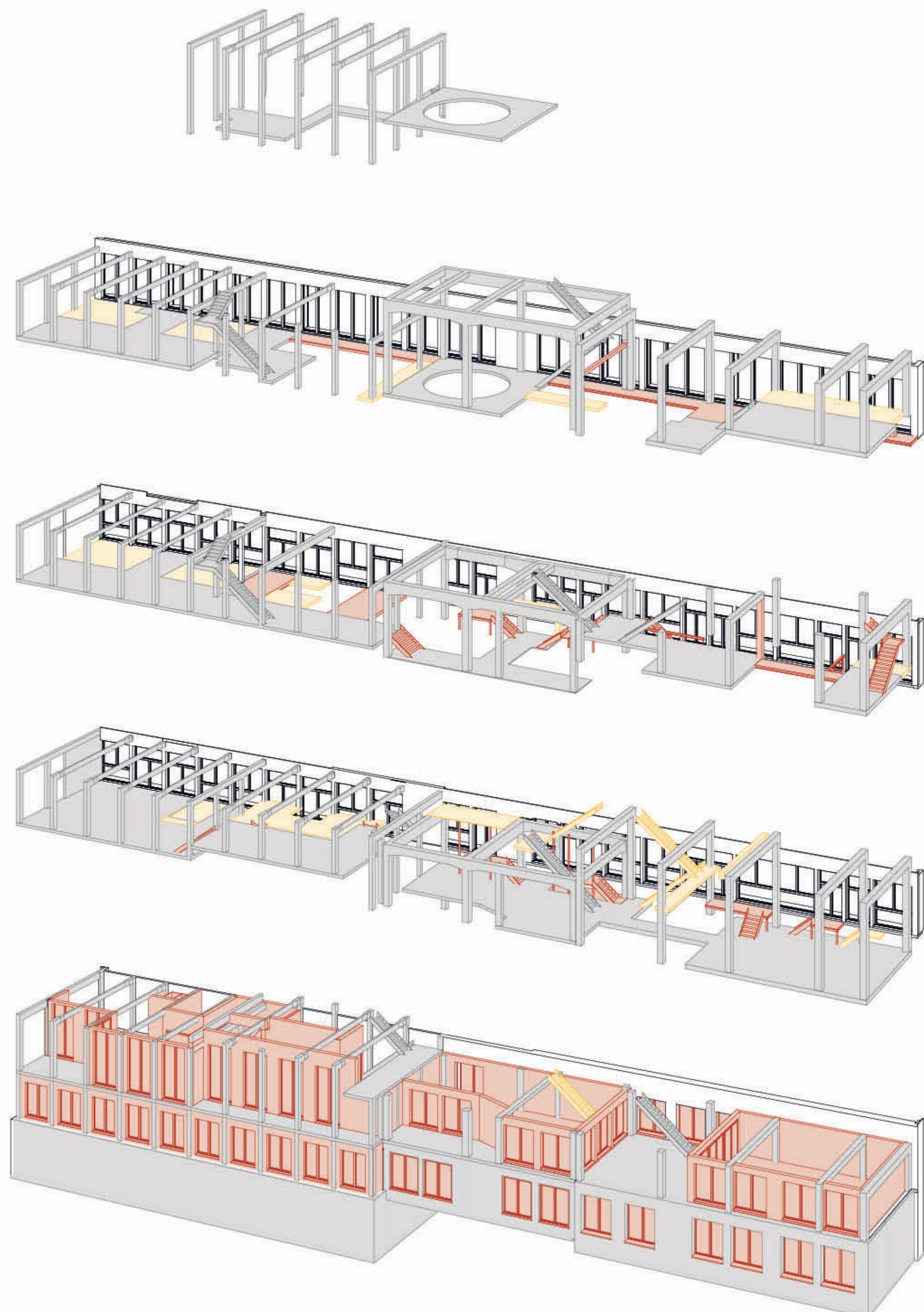
Schema Terrassenstruktur Bestand / Abbruch / Neu
