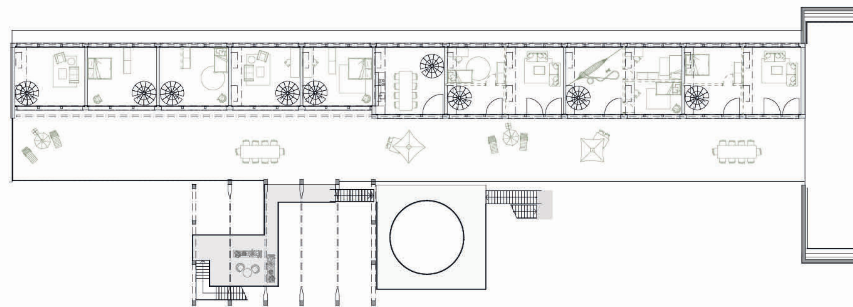
Grundriss 4.Obergeschoss (Aufstockung) | 1:200
