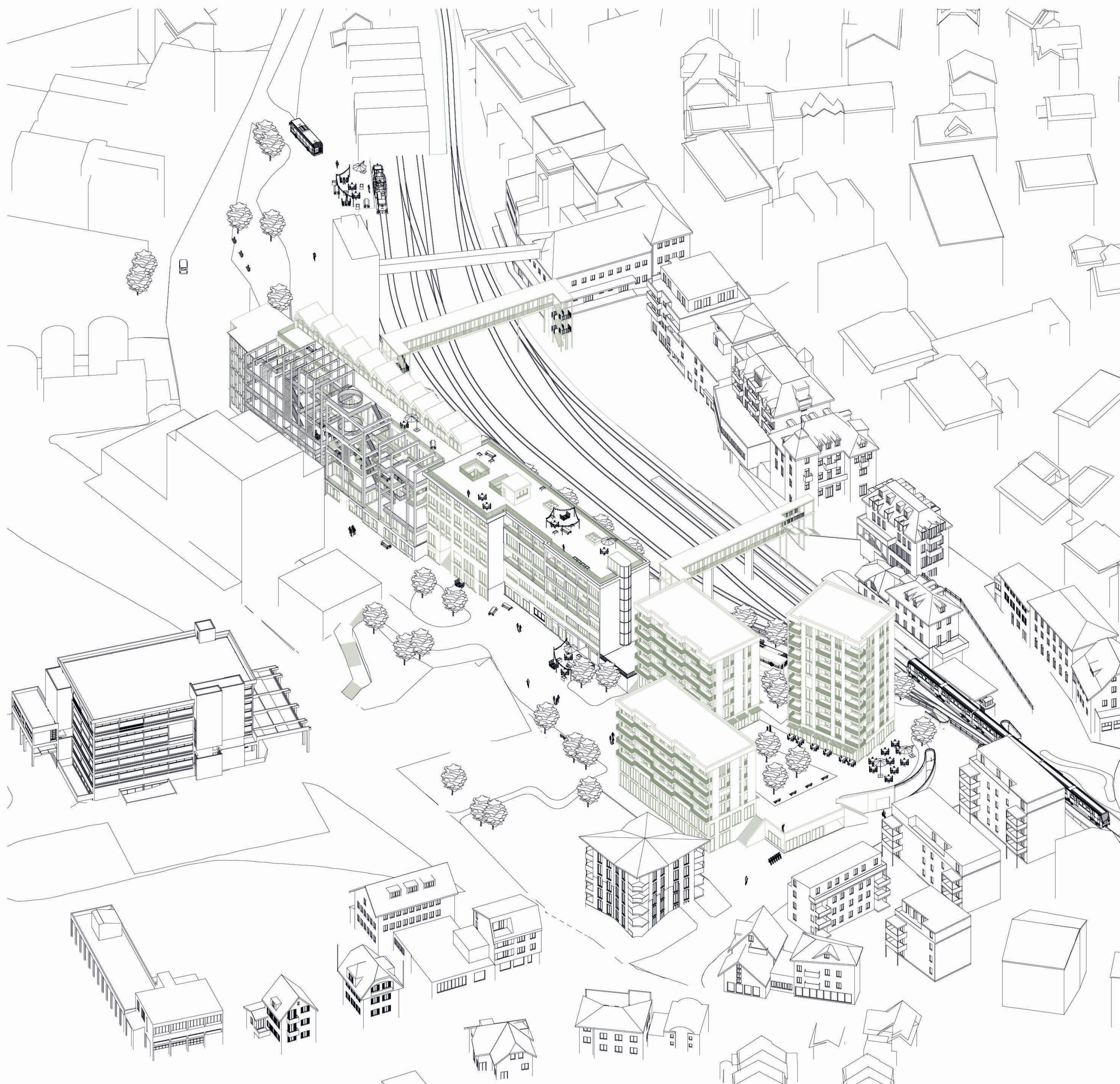
Schema Bestand / Abbruch / Neu
