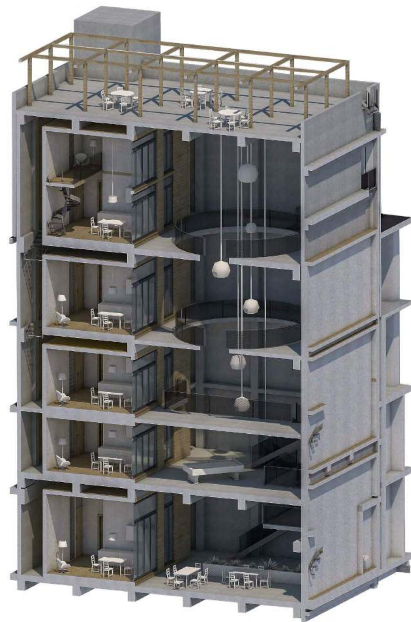
Axonometrie Fettpulverturm
