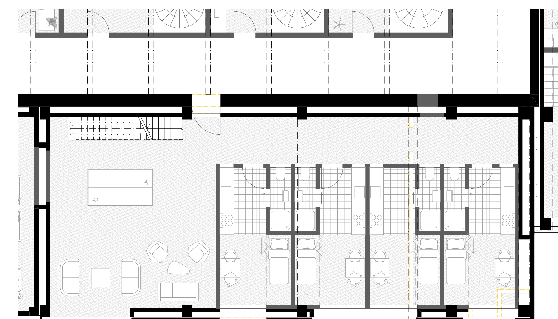
Erdgeschoss Niro 2 | Mst. 1:100
