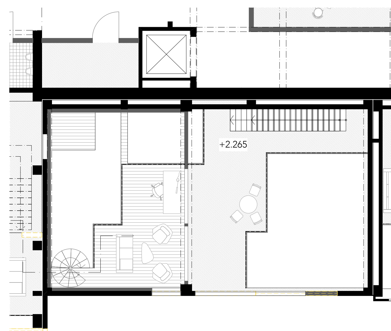
1. Obergeschoss Niro 1 | Mst. 1:100
