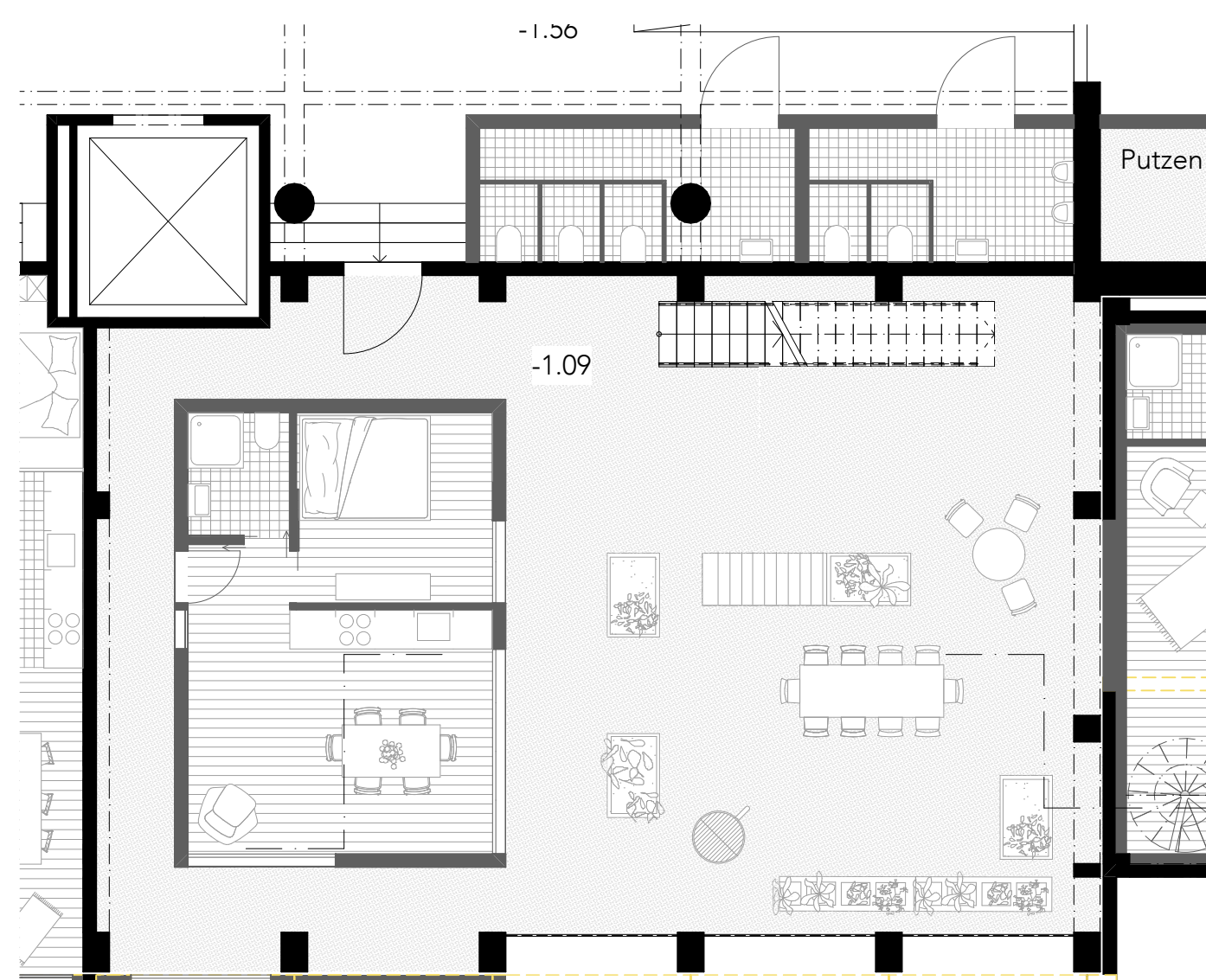
Erdgeschoss Fettpulverturm | Mst. 1:100
