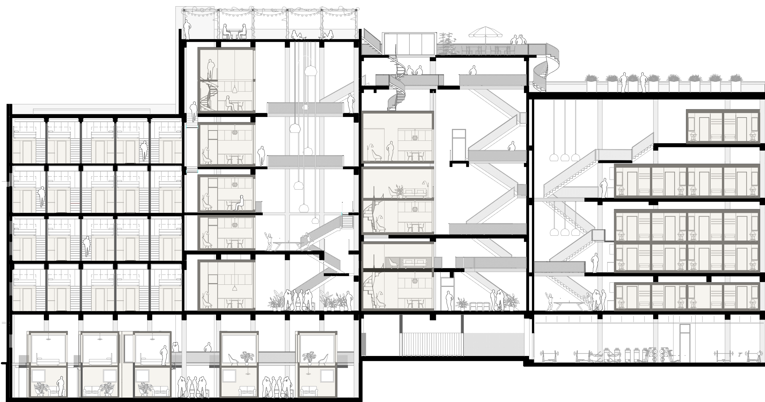
Längsschnitt Silos | Mst. 1:200
