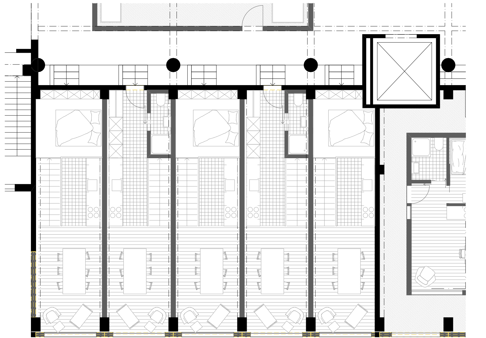
Erdgeschoss | Mst. 1:100
