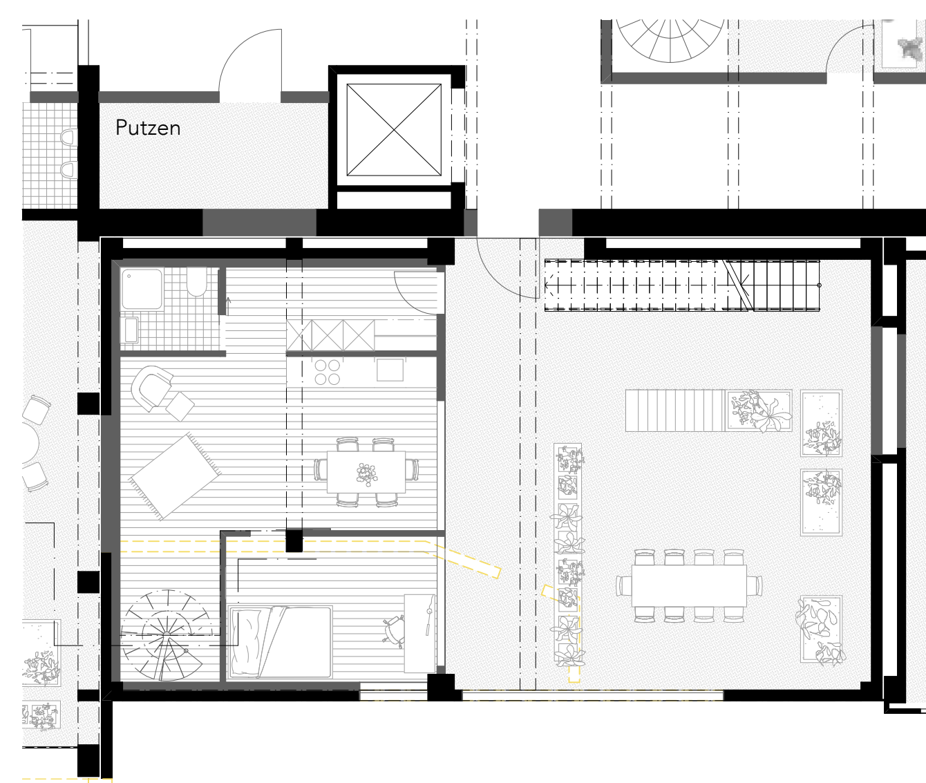
Erdgeschoss Niro 1 | Mst. 1:100
