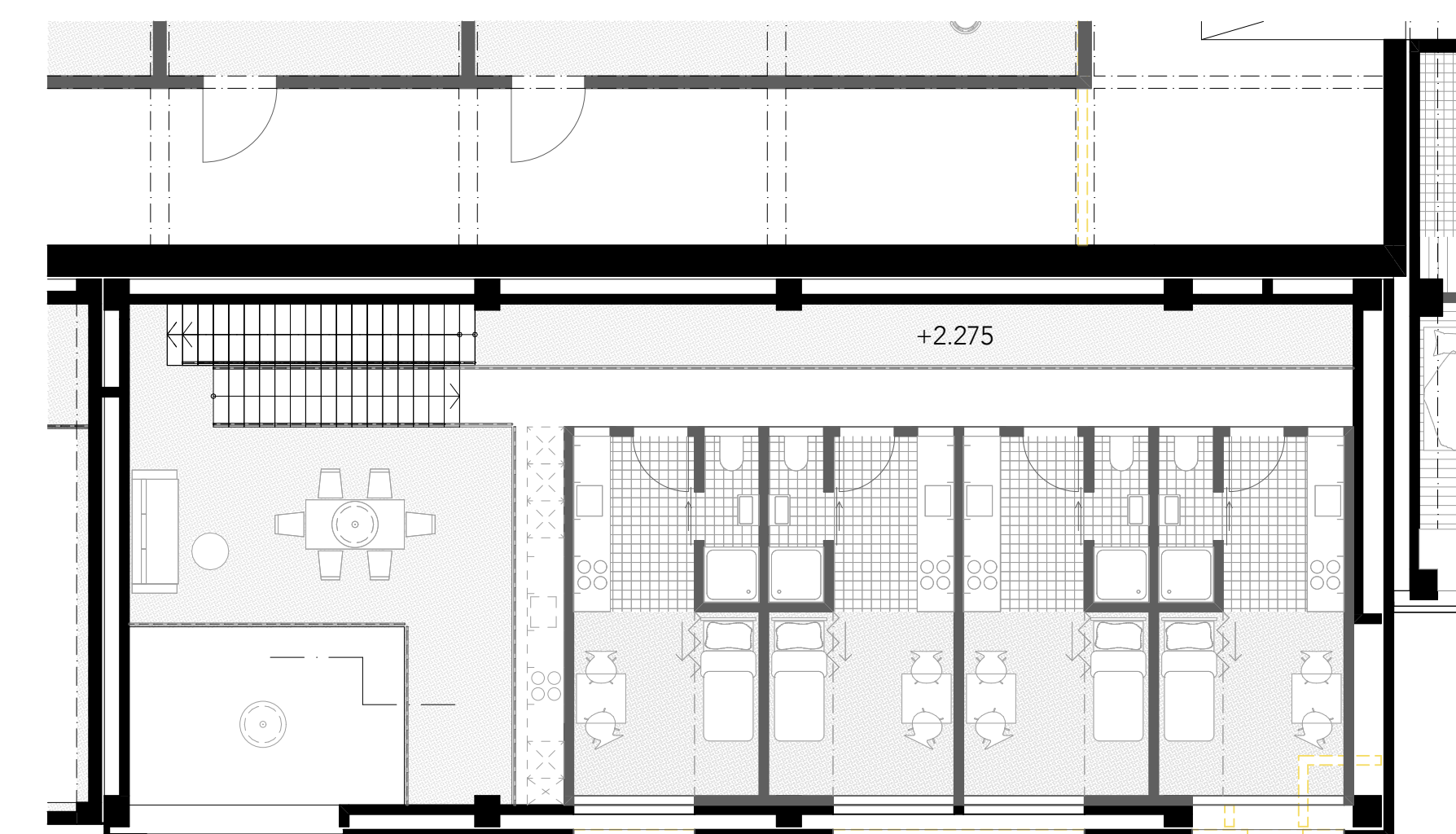
1. Obergeschoss Niro 2 | Mst. 1:100
