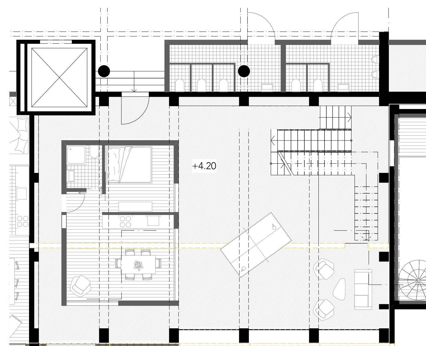
1. Obergeschoss Fettpulverturm | Mst. 1:100
