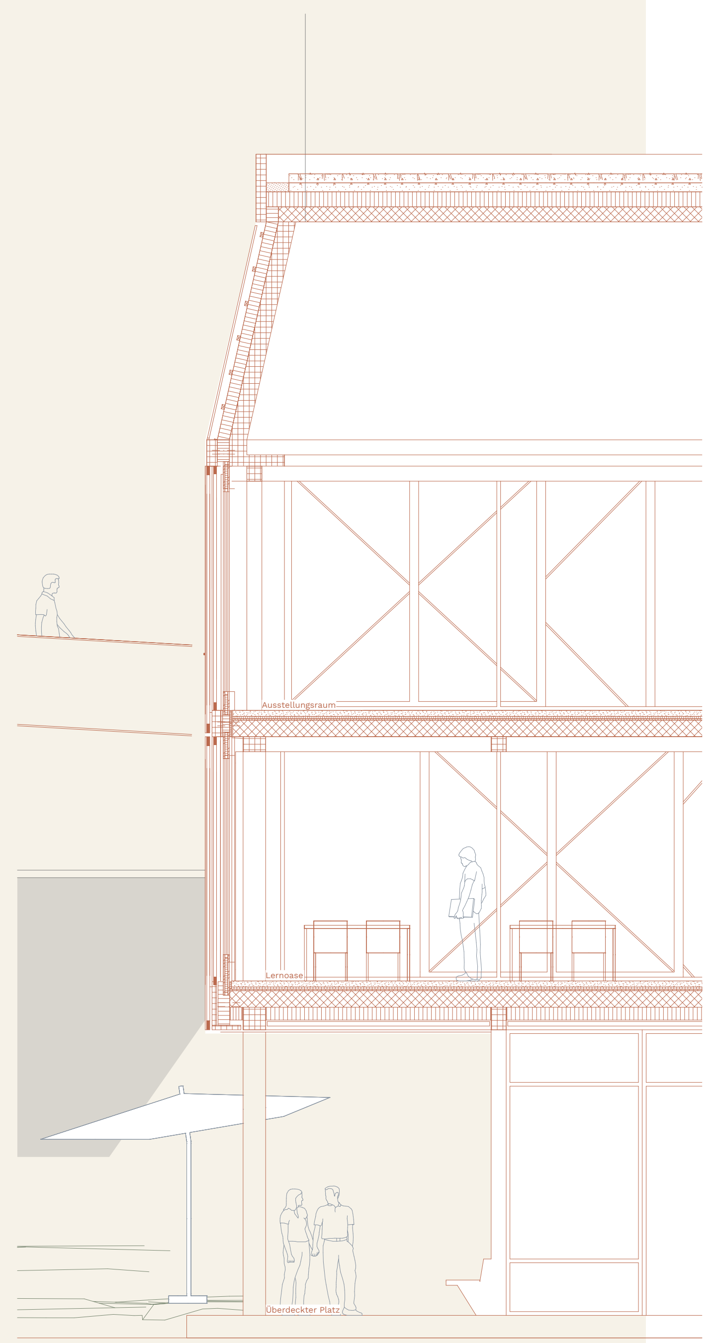
Fassadenschnitt Neubau | 1:50
