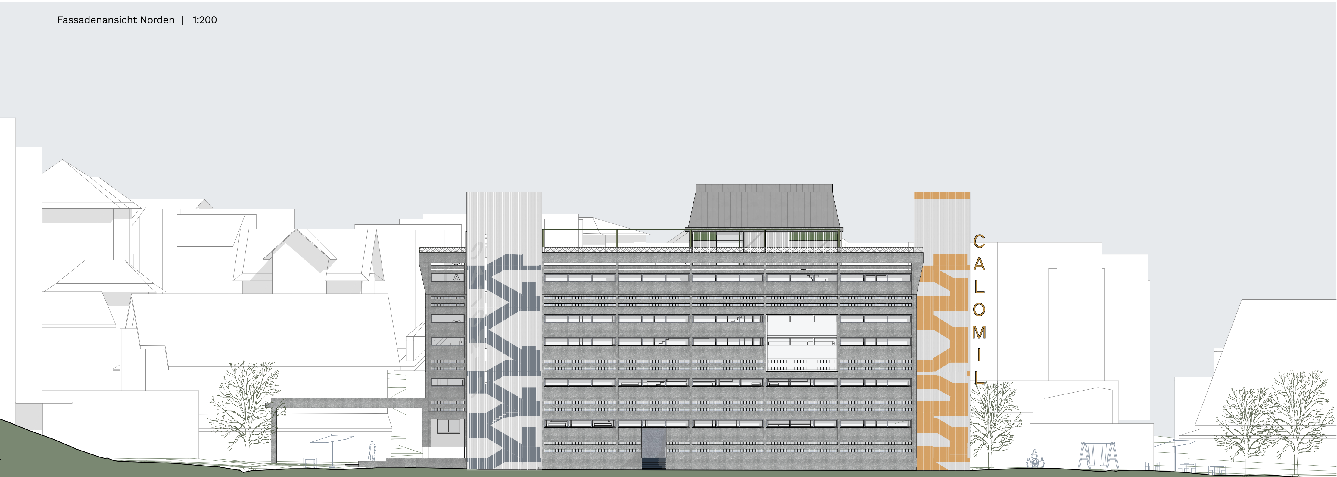
Fassadenansicht Norden | 1:200
