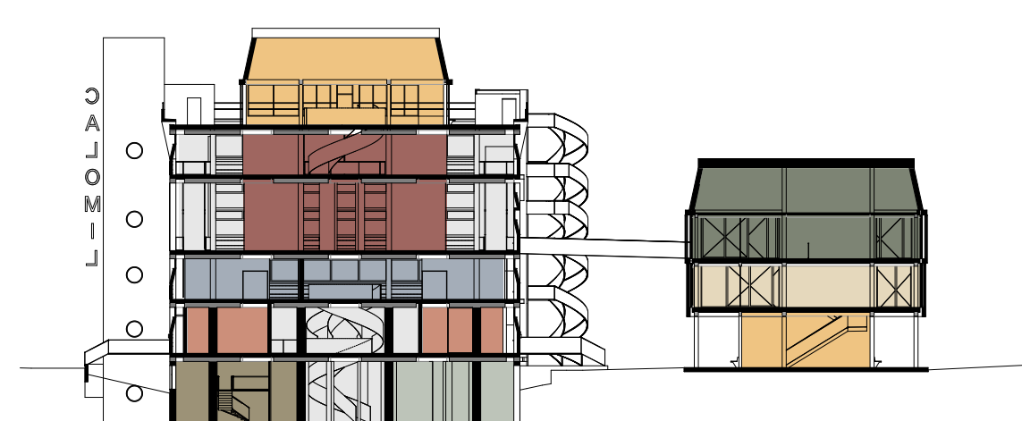
Schemaplan - Querschnitt Calomil | 1:500
