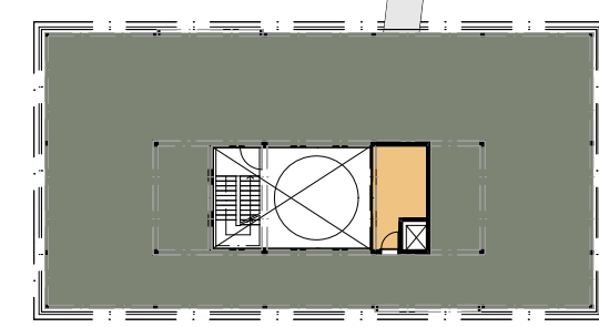
Schemaplan - 2. Obergeschoss | 1:500
