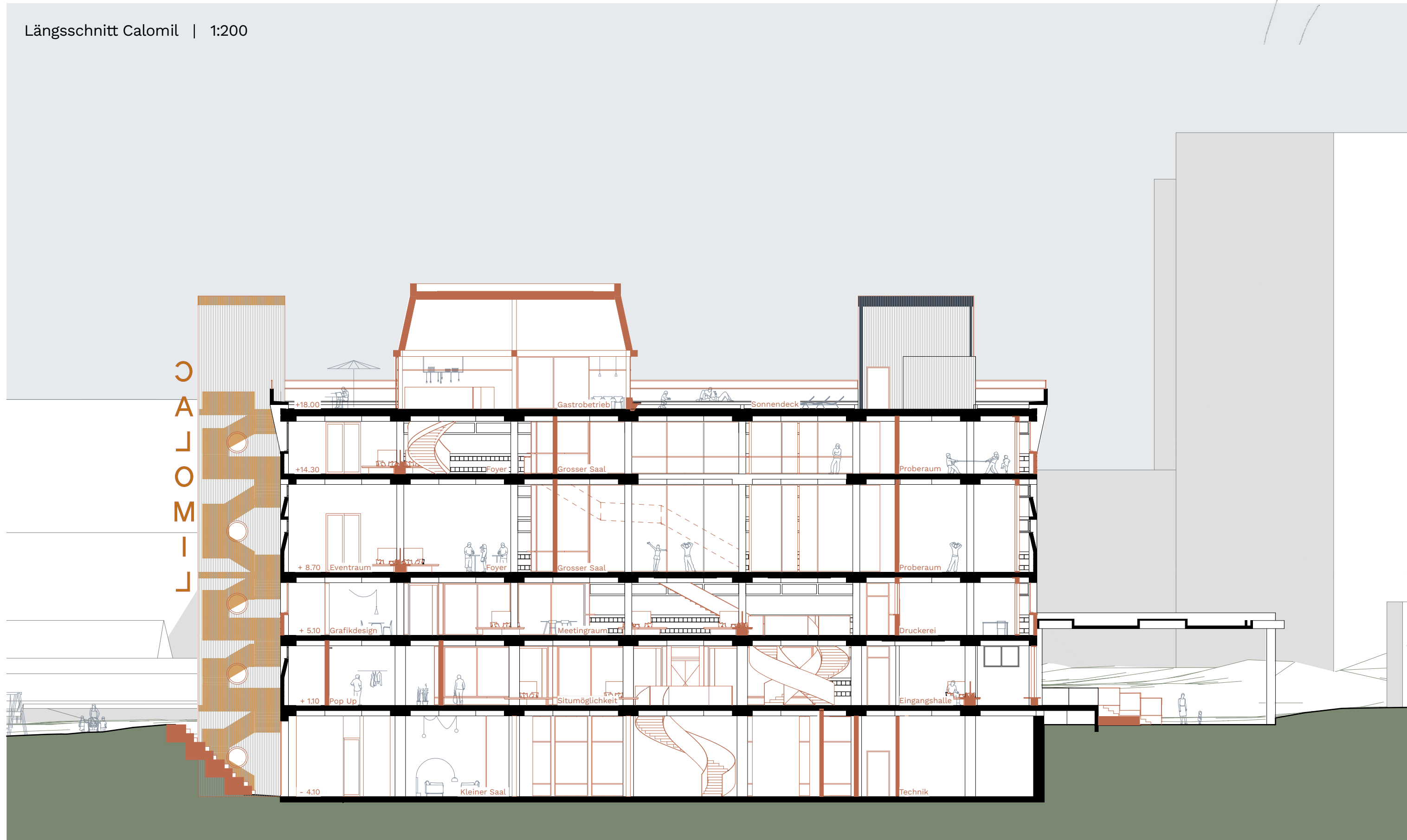
Längsschnitt Calomil | 1:200
