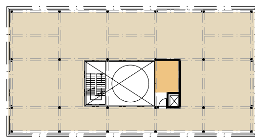
Schemaplan - 1. Obergeschoss | 1:500
