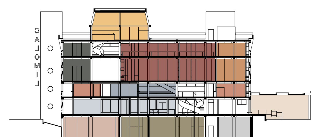
Schemaplan - Längsschnitt Calomil | 1:500
