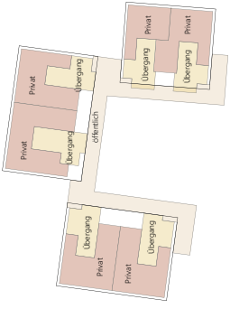
Schema Zonierung
