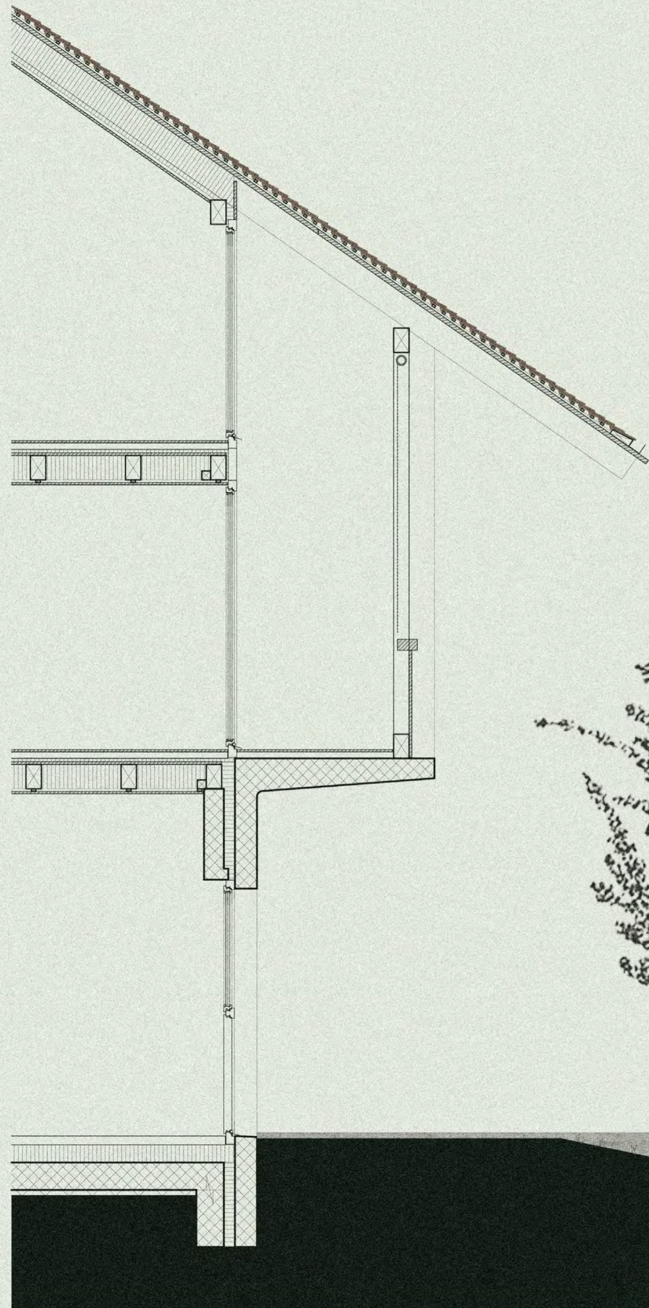
Fassadenschnitt Stallgebäude
