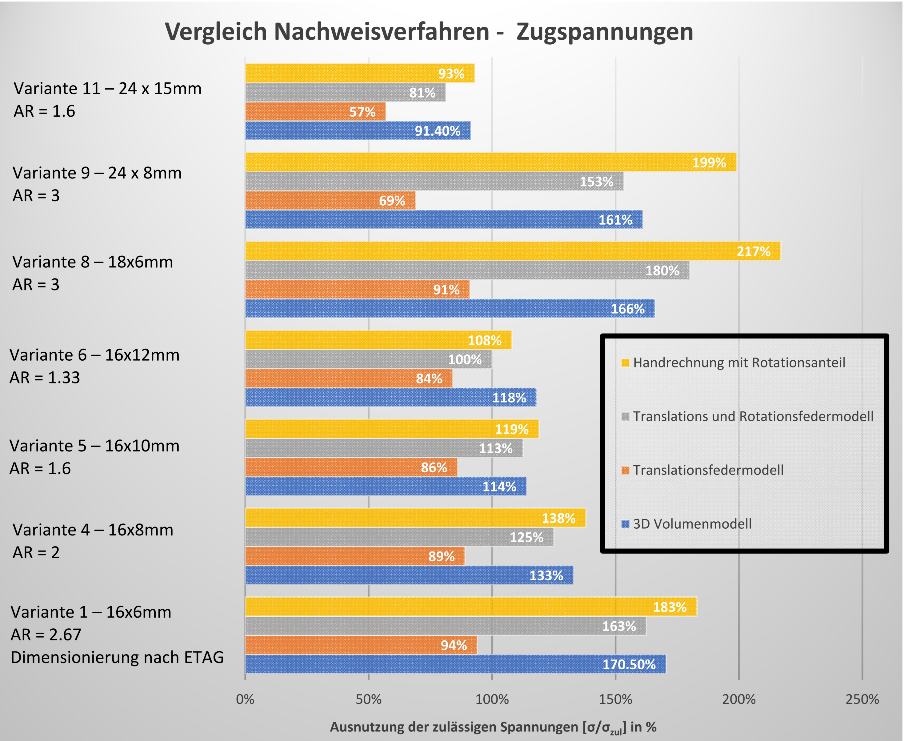
Abb. 10: Vergleich der Nachweisverfahren Bezüglich deren Grad der Nachweiserfüllung der Zugspannungen im Silikon
