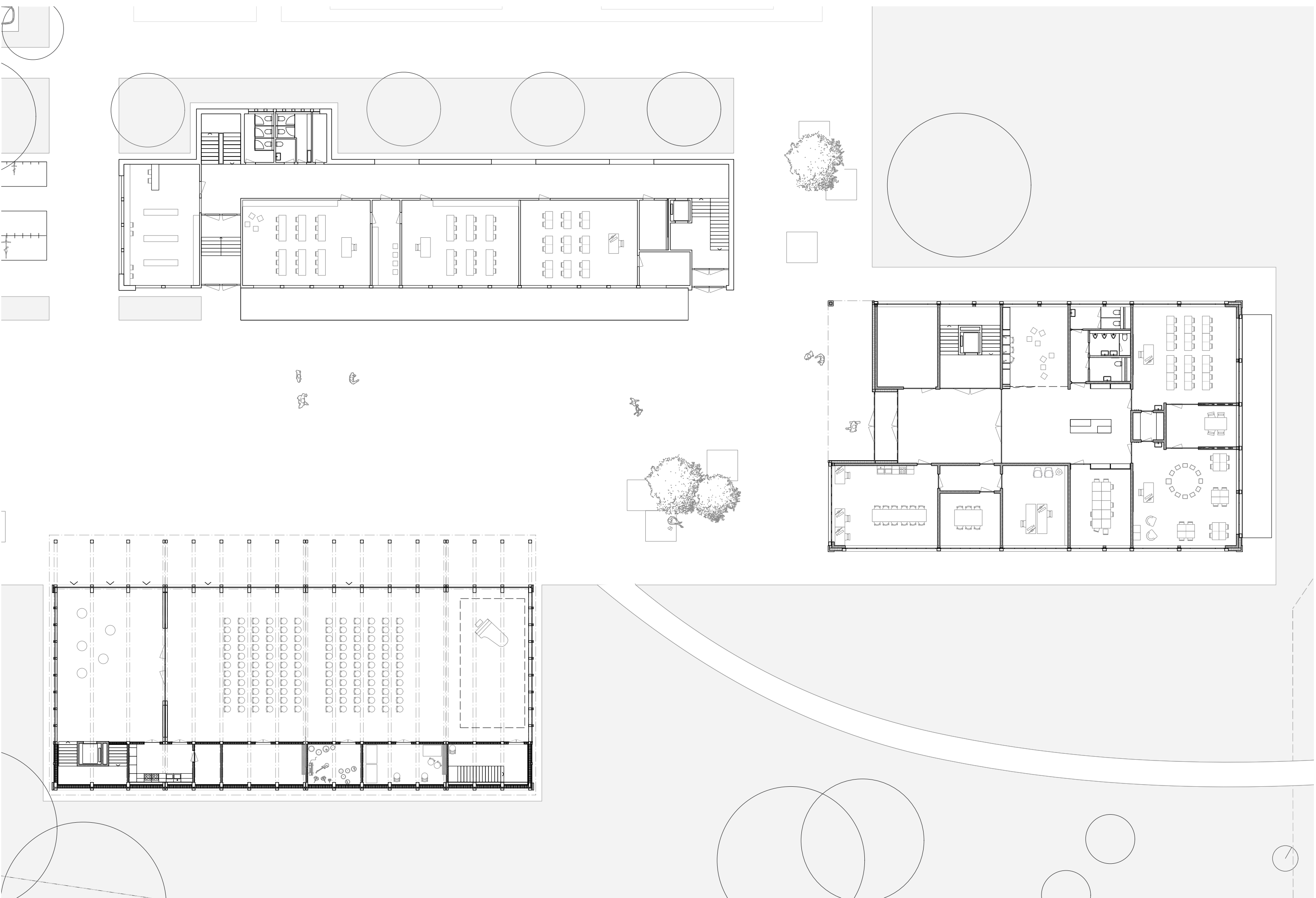
Grundriss Erdgeschoss
