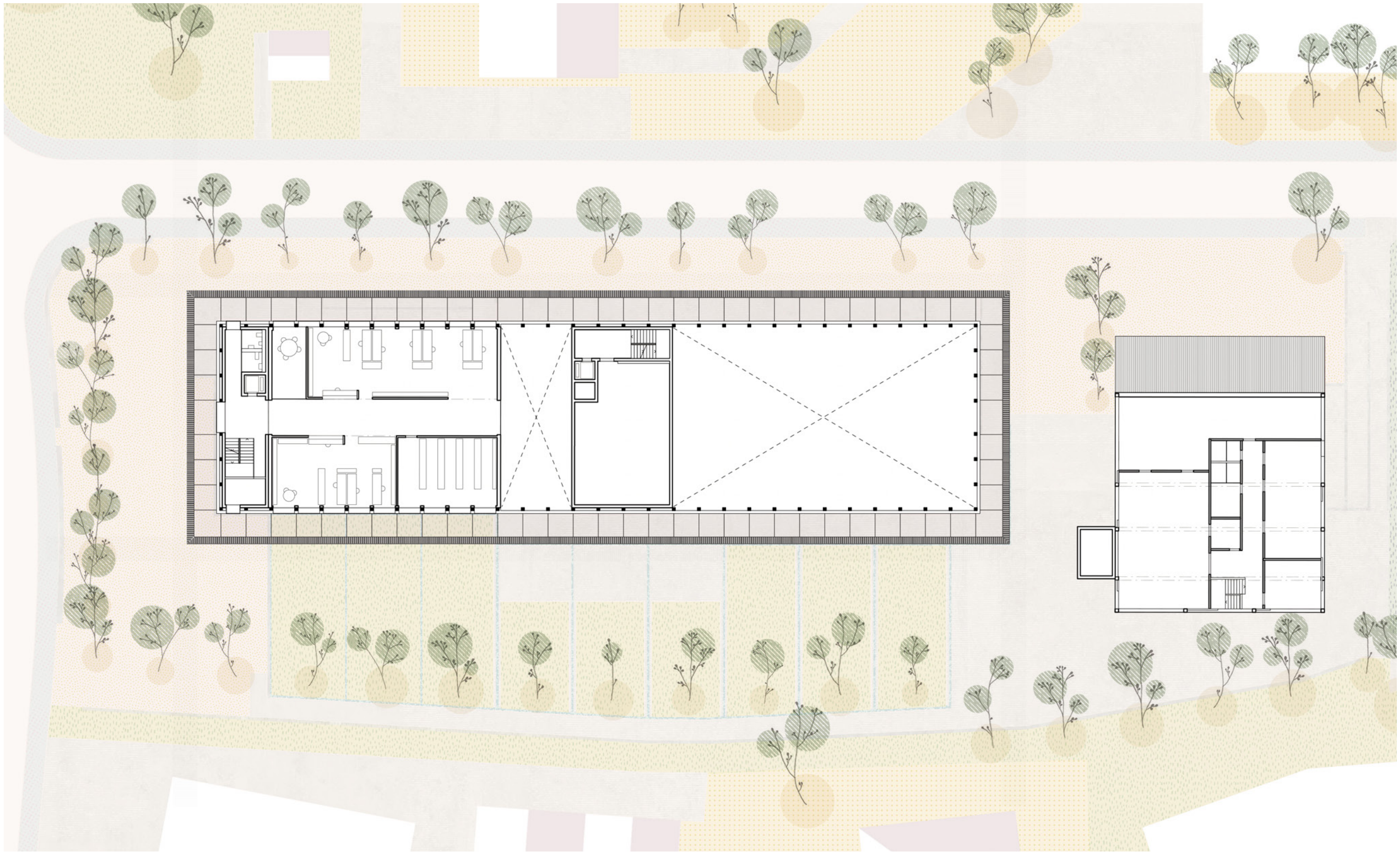
1. Obergeschoss
