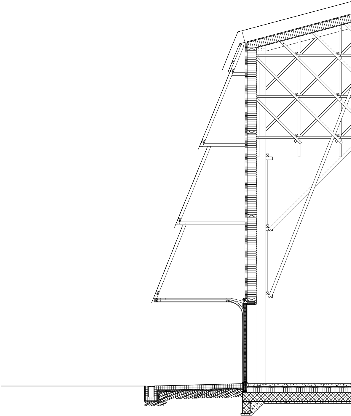
Fassadenschnitt Aula
