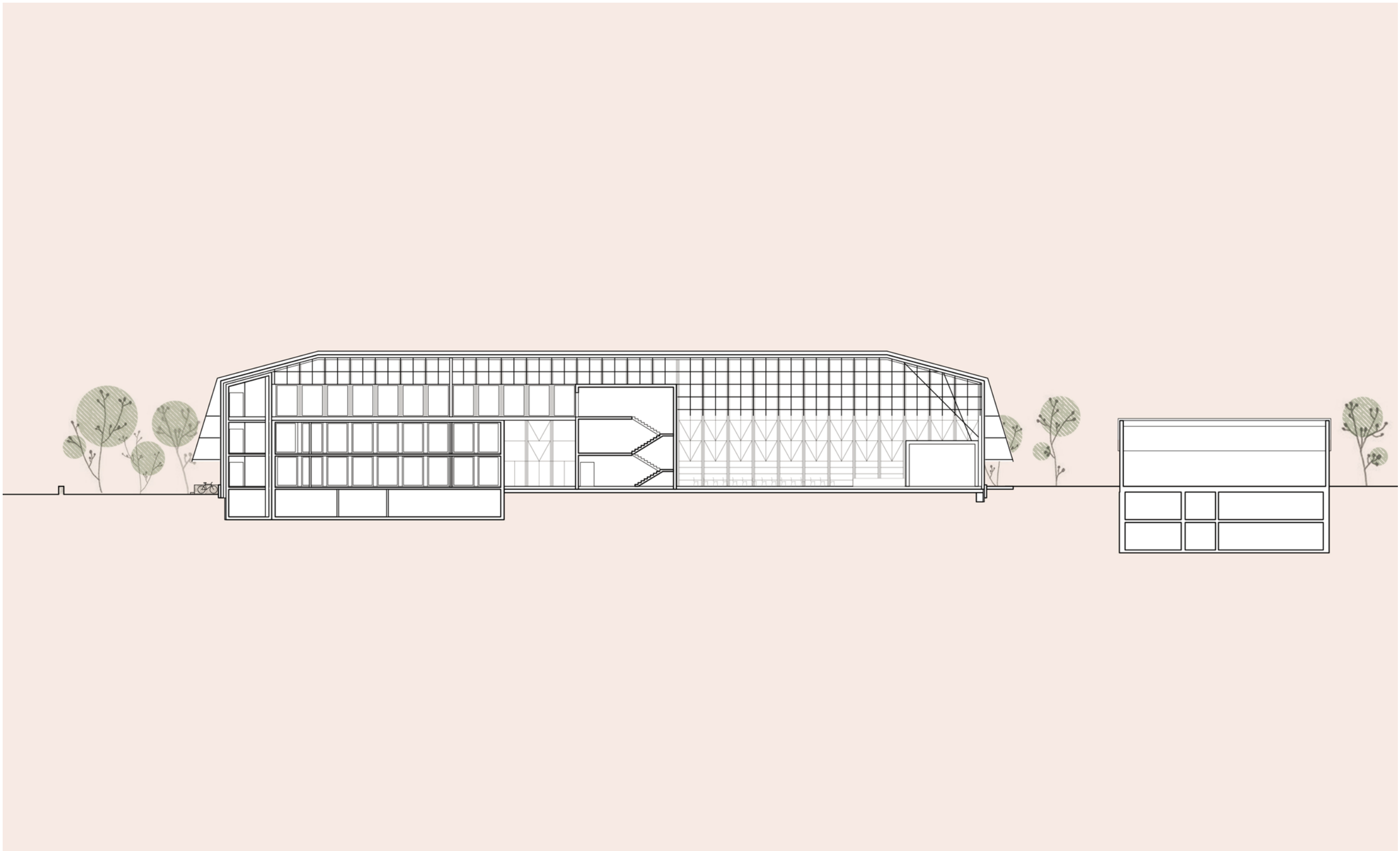
Längsschnitt 1
