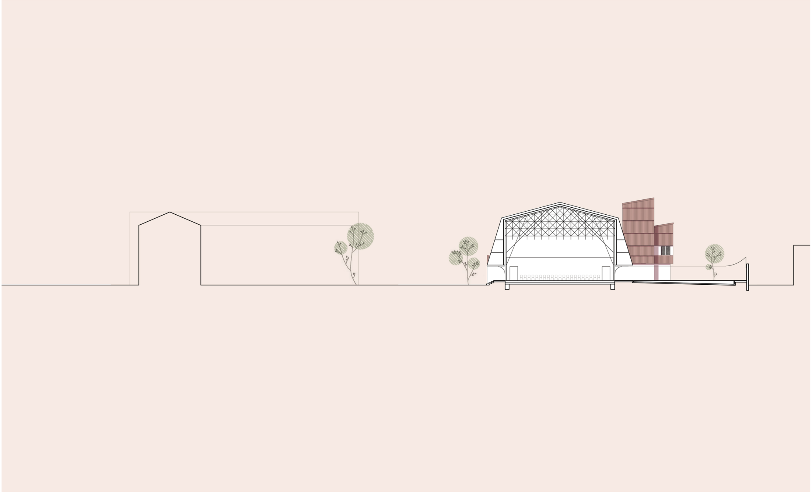
Querschnitt Aula
