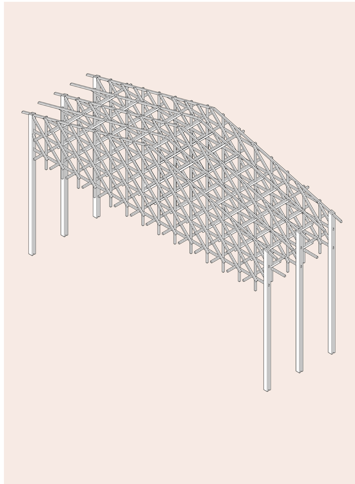
Tragwerk - Aussteifung über Aula
