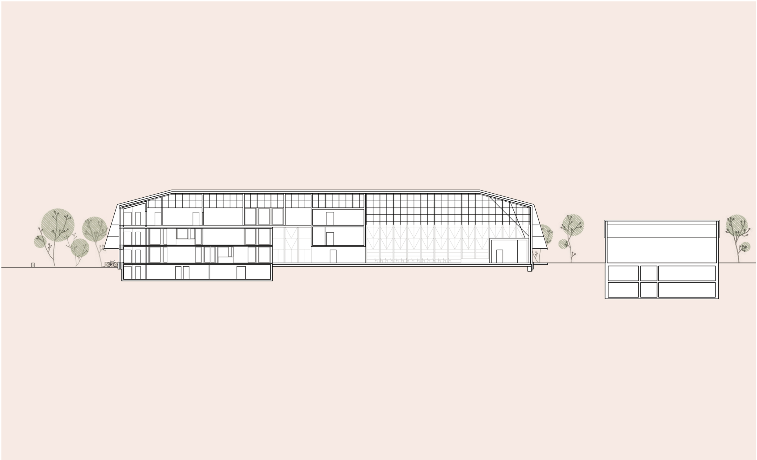
Längsschnitt 2
