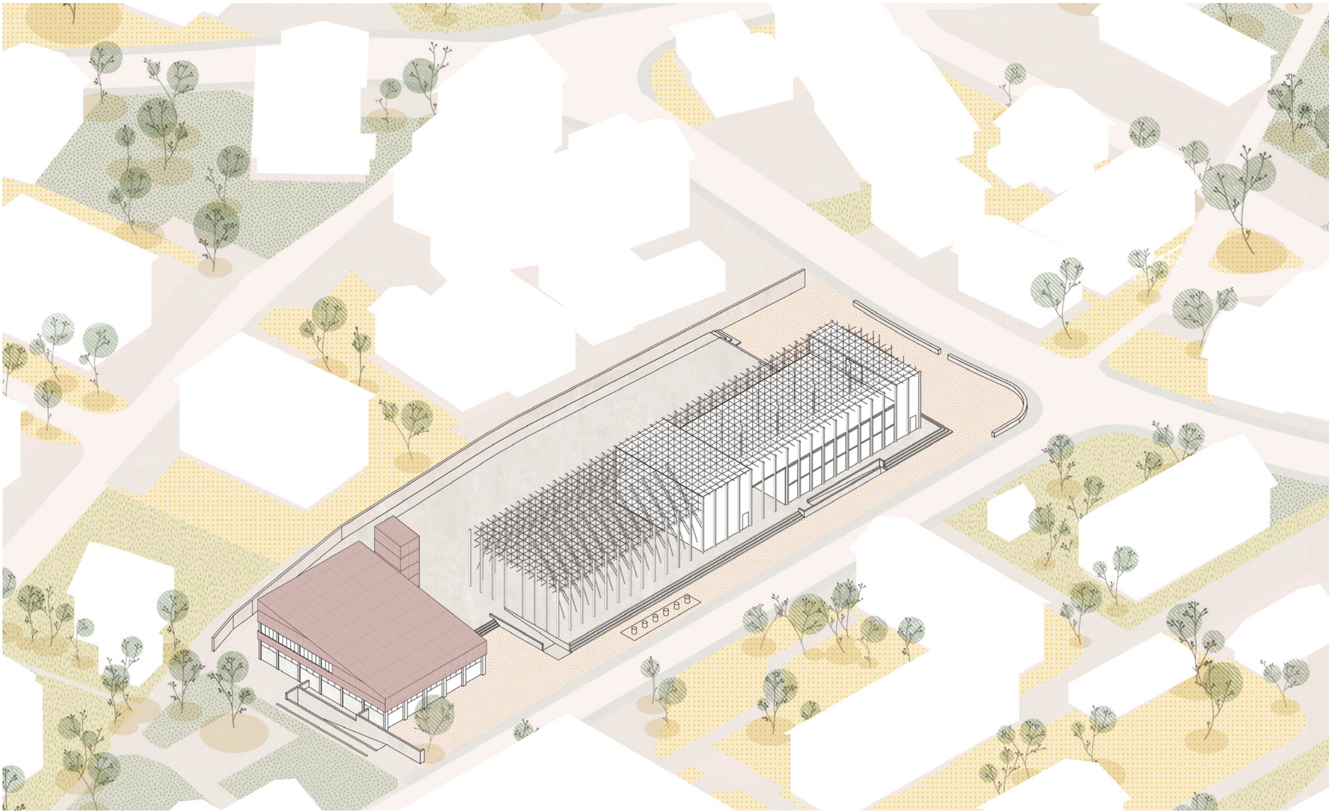
Axonometrie - Gitterwerk
