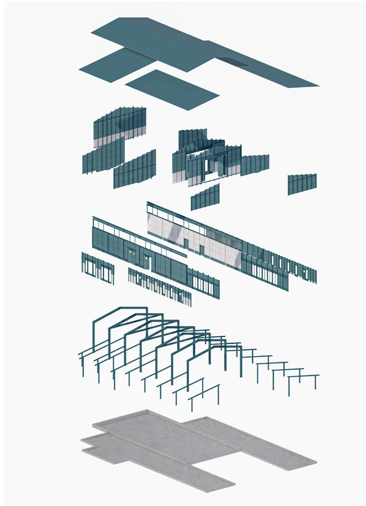
Tragwerkskonzept
