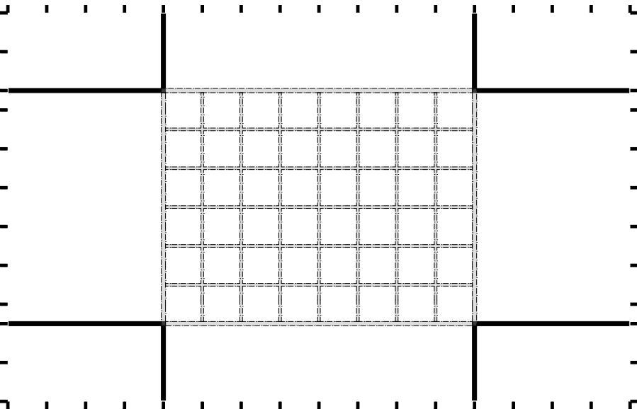
Grundriss
