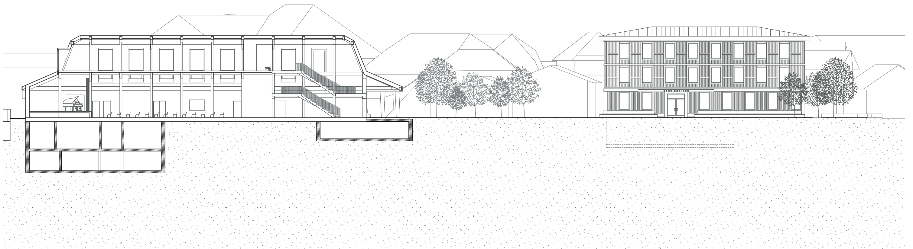
Längsschnitt Aula
