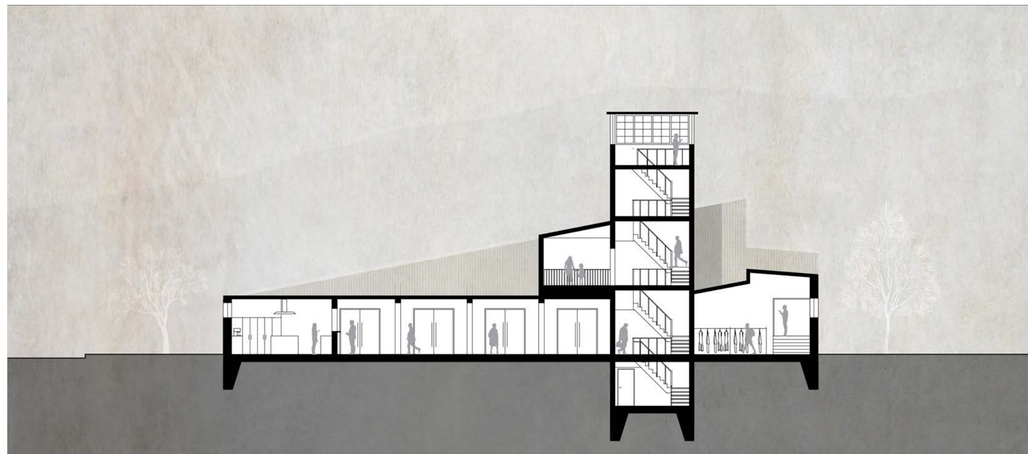
Querschnitt durch Foyer und Aussichtsturm
