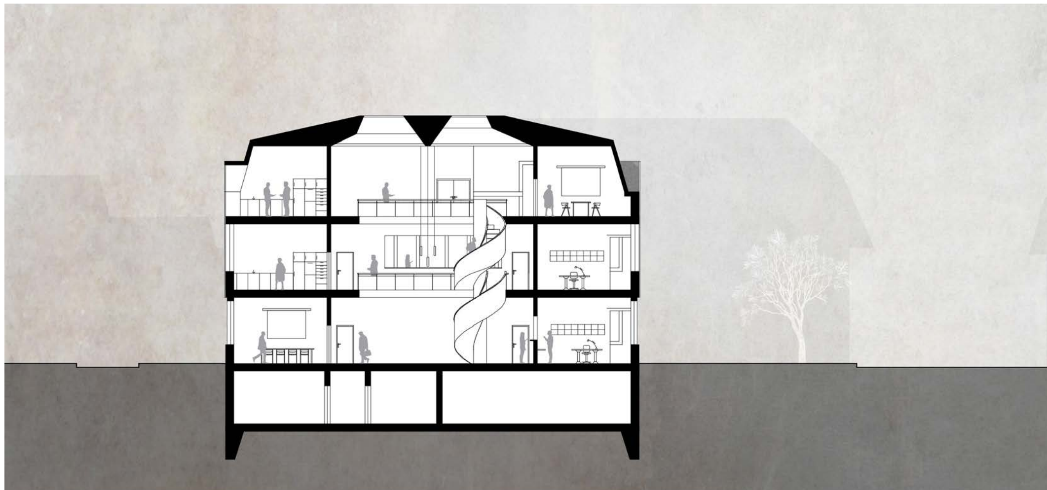
Querschnitt Verwaltungsgebäude vom Dorfplatz zur Hauptstrasse
