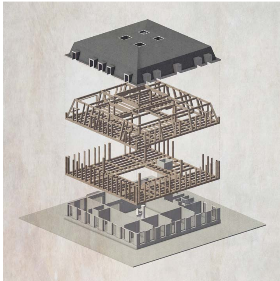
Konstruktionsaxonometrie der aufgeständerten Holzkonstruktion
