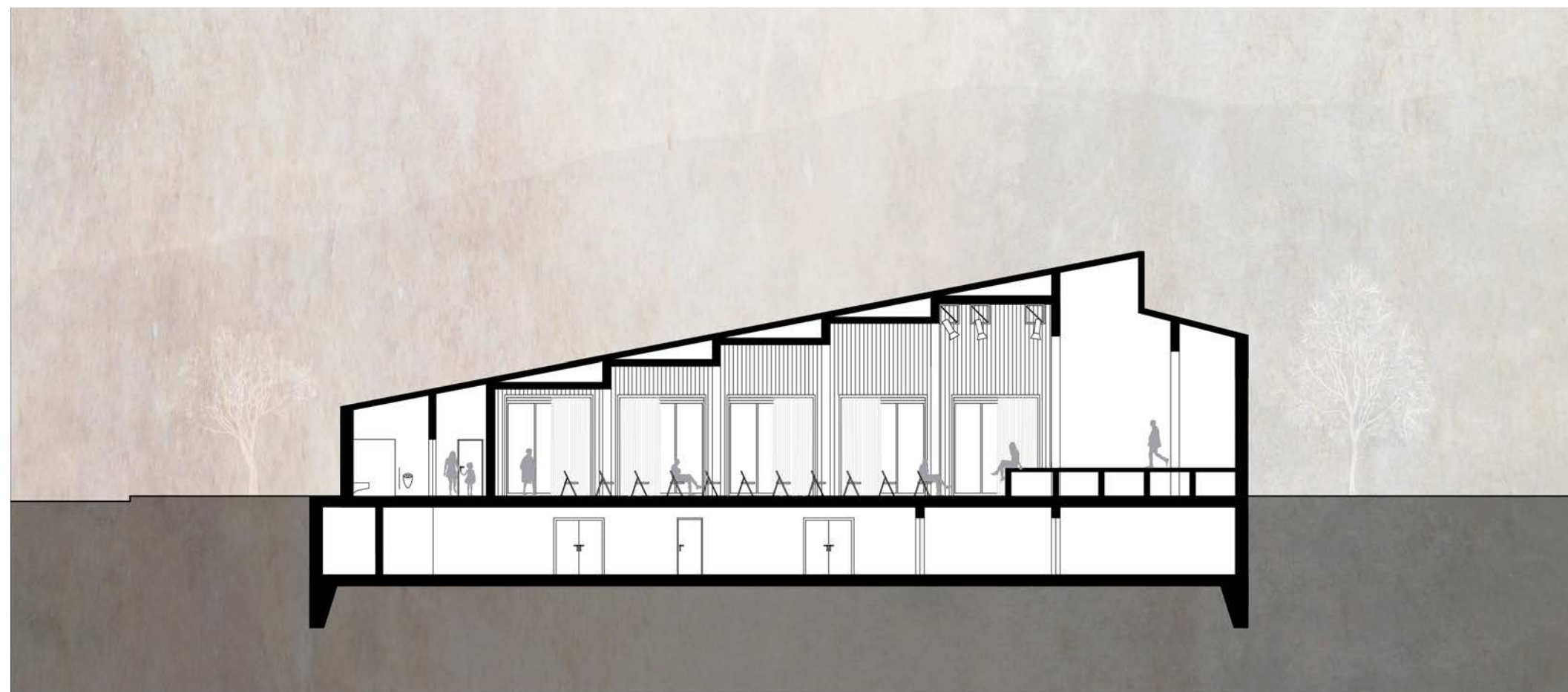
Konstruktionsschnitt Aula mit Bestand und Anbau
