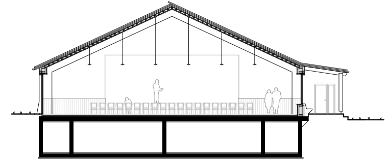
Querschnitt
