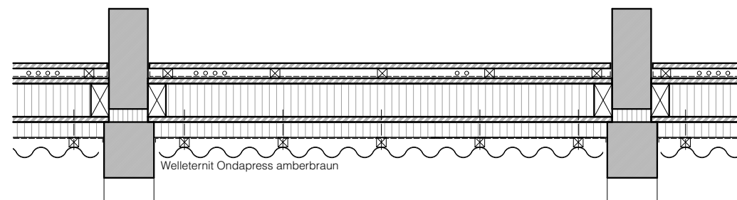
Horizontalschnitt durch Brüstung
