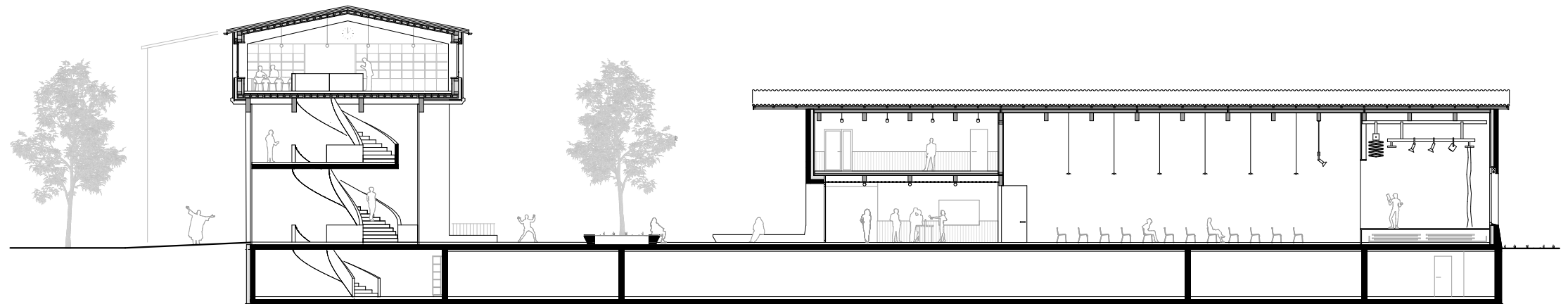
Schnitt Ensemble
