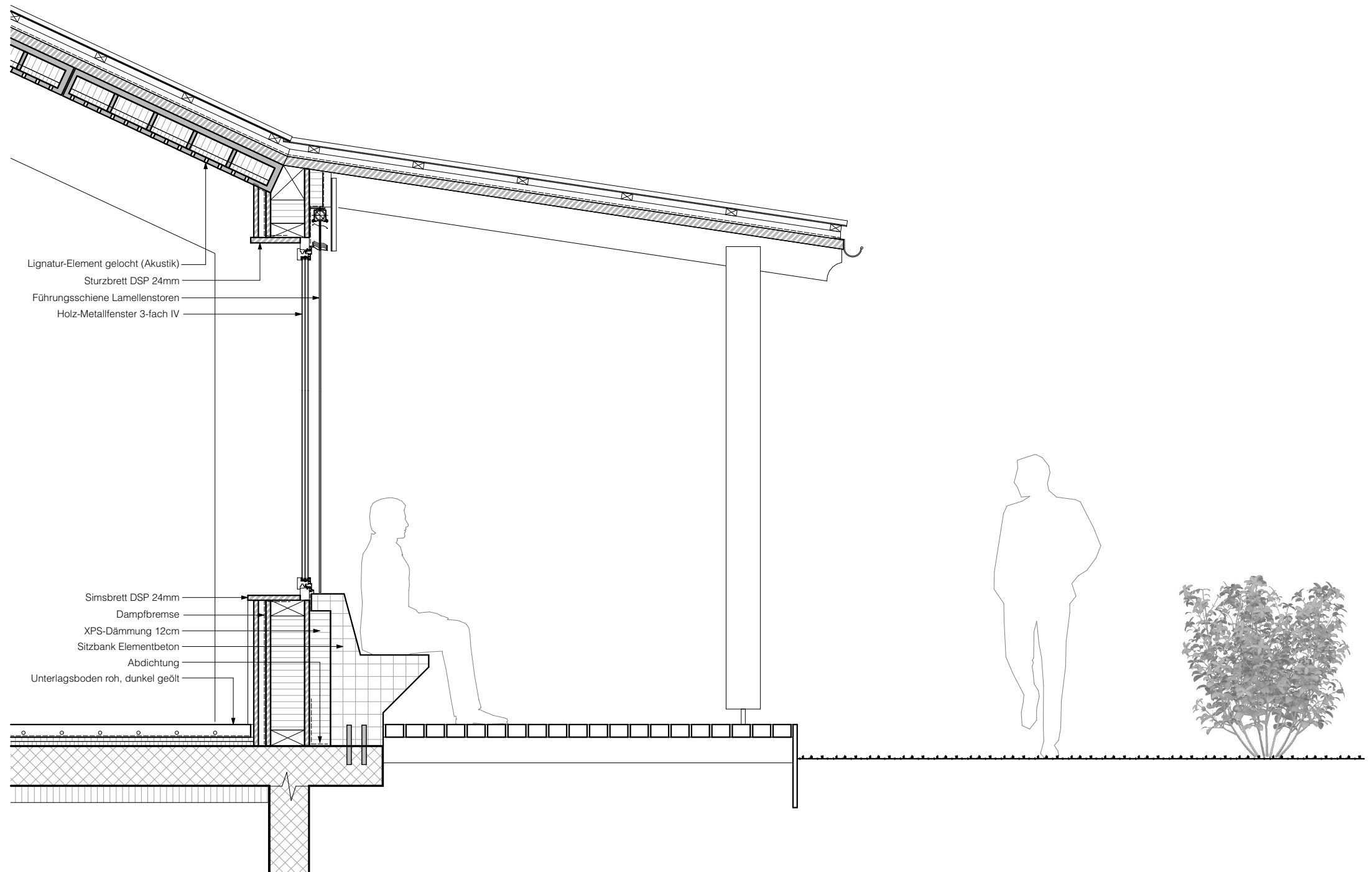
AULA - KONSTRUKTION
