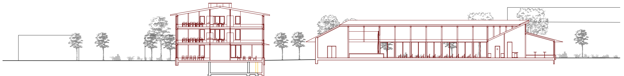
Schnitt durch Schulhaus- und Aulagebäude
