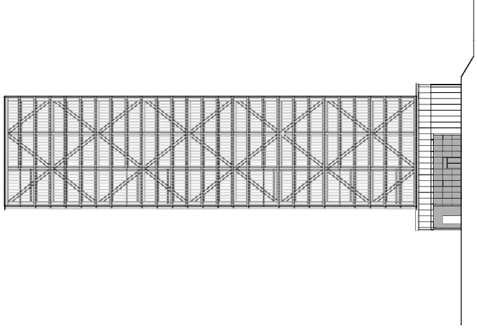
Fassade Ost
