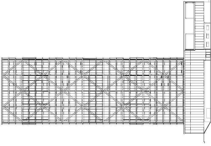
Fassade Nord
