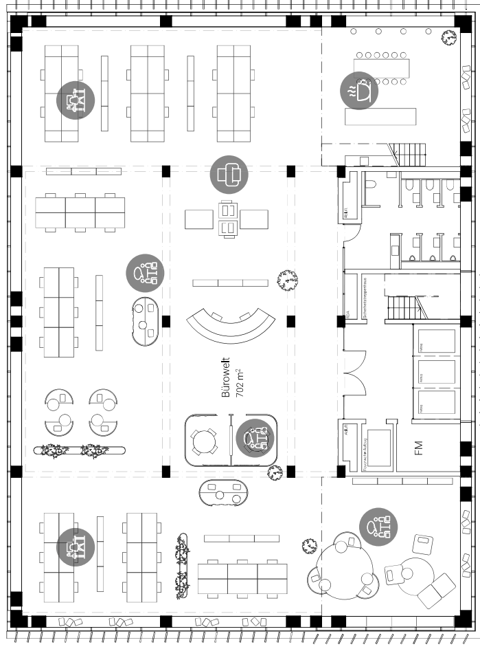
Ebene 1
