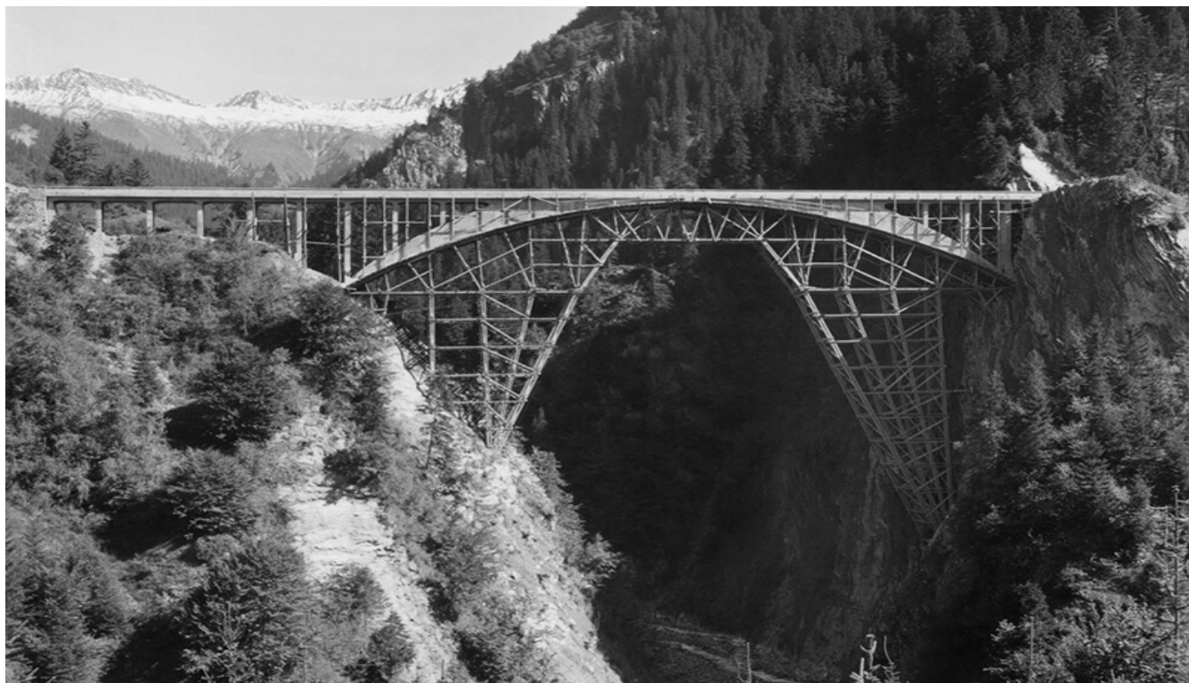
Salginatobelbrücke von Robert Maillard • Leegerüst von Richard Coray • 1930
